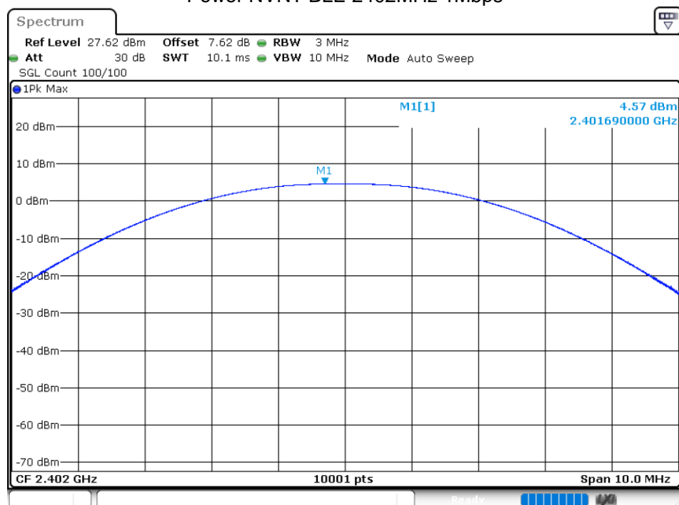
Power NVNT BLE 2402MHz 1Mbps
