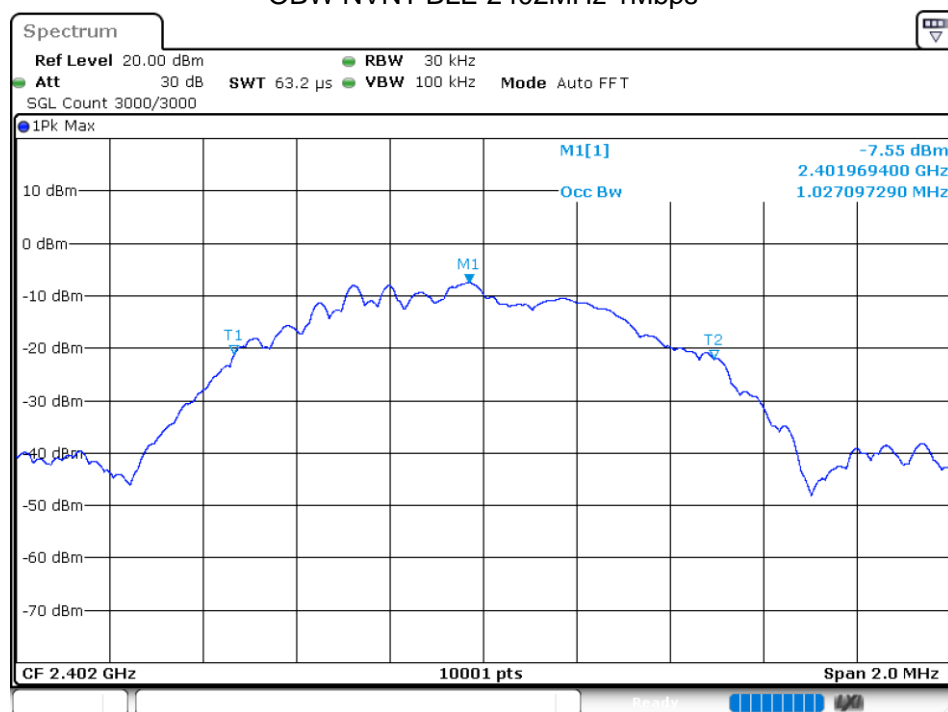
OBW NVNT BLE 2402MHz 1Mbps
