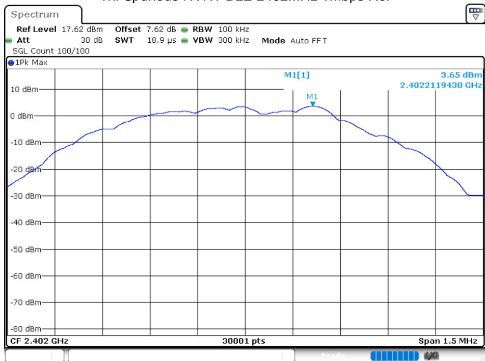
Tx. Spurious NVNT BLE 2402MHz 1Mbps Ref
