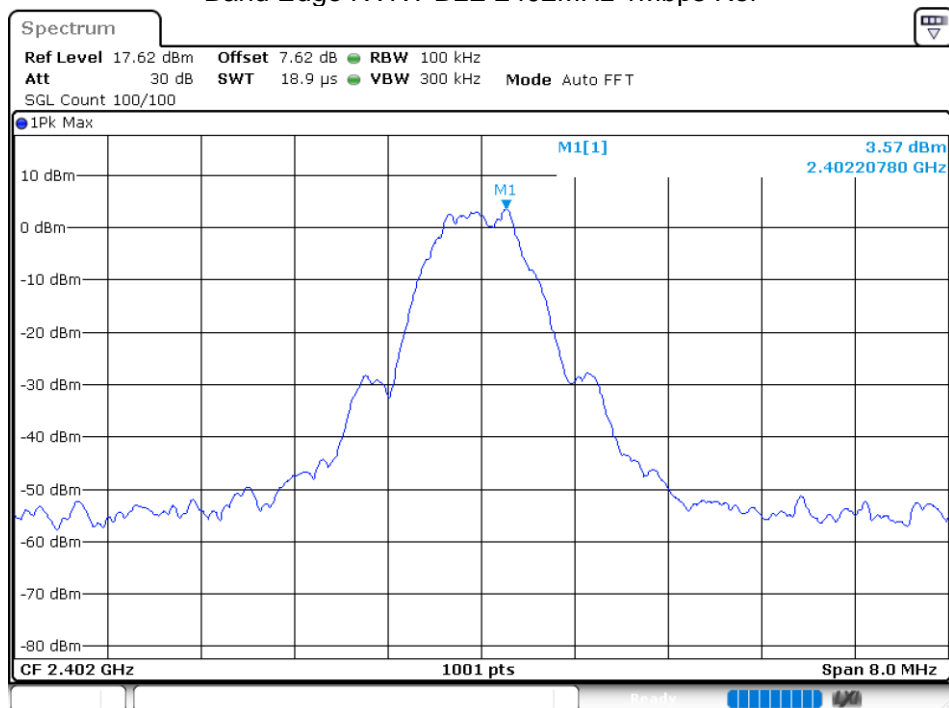
Band Edge NVNT BLE 2402MHz 1Mbps Ref
