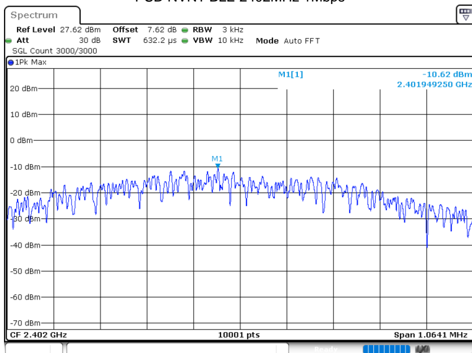
PSD NVNT BLE 2402MHz 1Mbps
