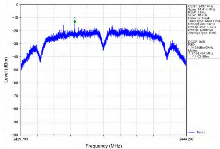
802.11b_MCH_2437MHz_Ant1 (SISO)_NTNV
