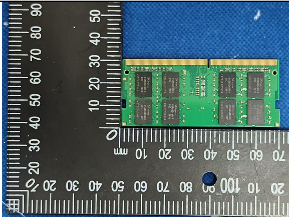
EUT Photo
