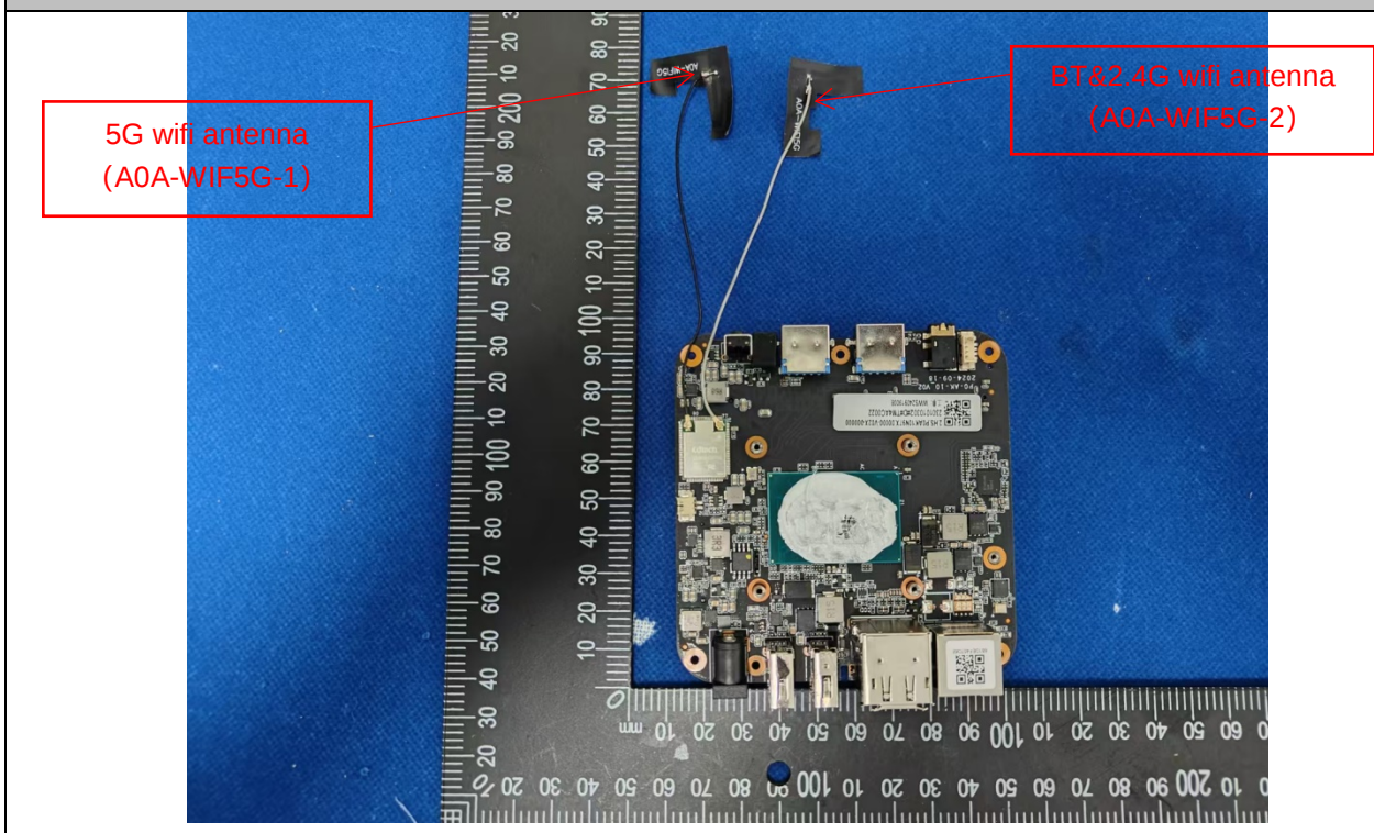
EUT Photo
