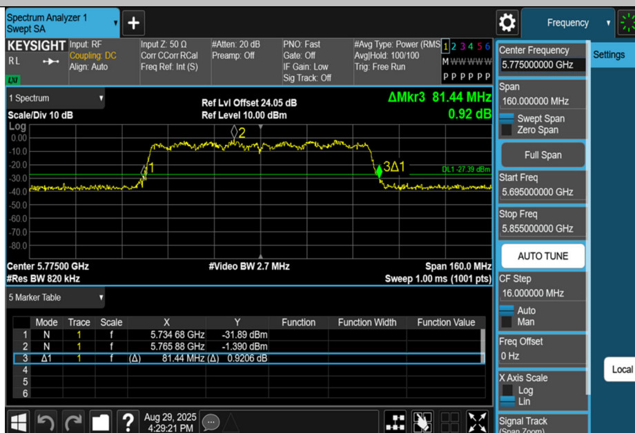
11AC80SISO-Ant1-5775
