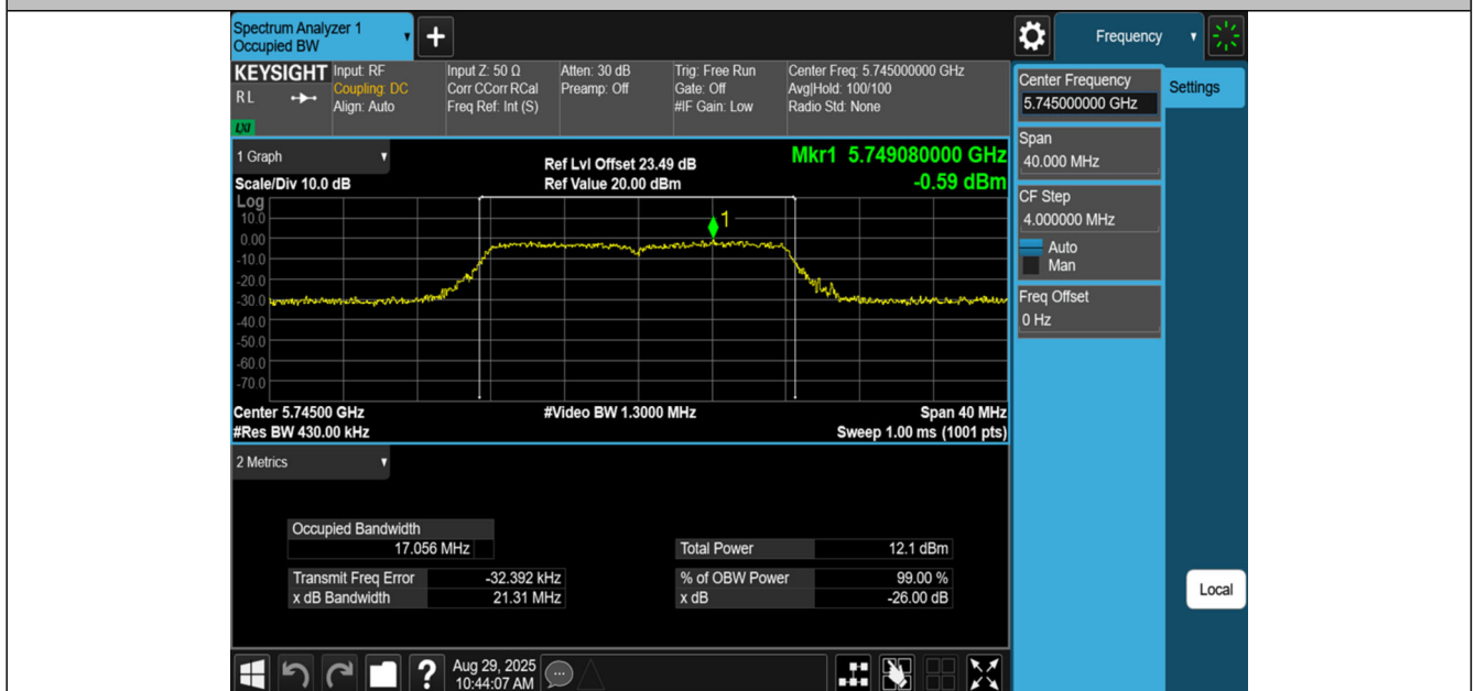
11A-Ant1-5745
