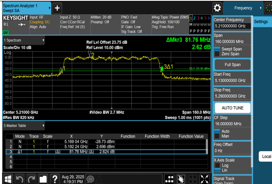
11AC80SISO-Ant1-5210
