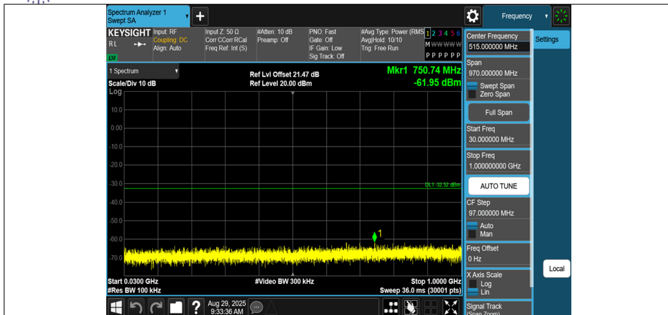
11G-Ant1-2462-30~1000-PASS
