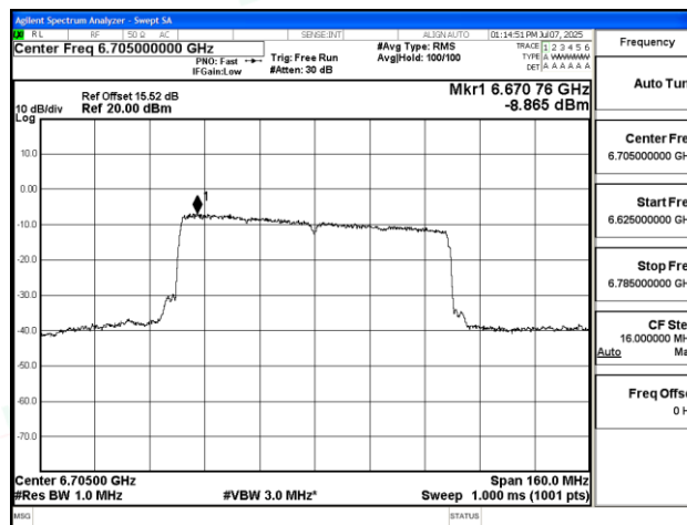
11AX80SISO-Ant1-6705-PASS
