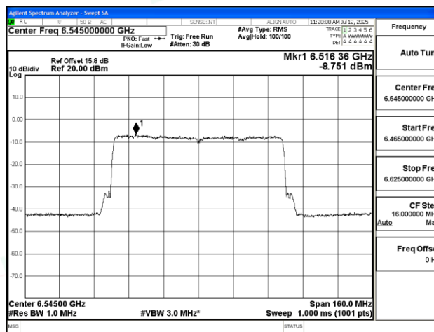
11AX80SISO-Ant1-6545-PASS
