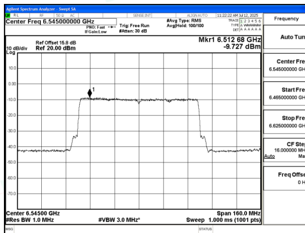
11AX80SISO-Ant2-6545-PASS
