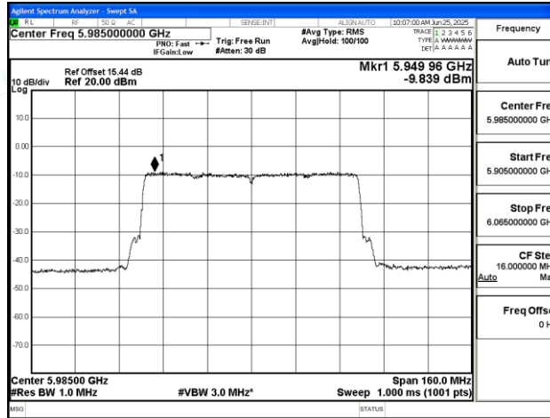
11AX80SISO-Ant2-5985-PASS
