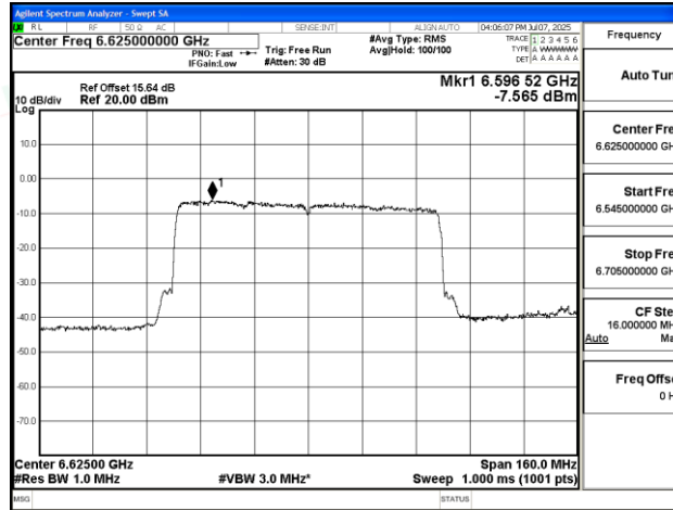
11AX80SISO-Ant1-6625-PASS
