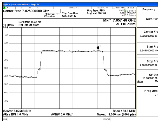
11AX80SISO-Ant2-7025-PASS
