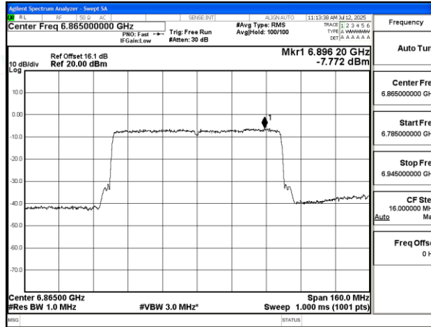
11AX80SISO-Ant1-6865-PASS
