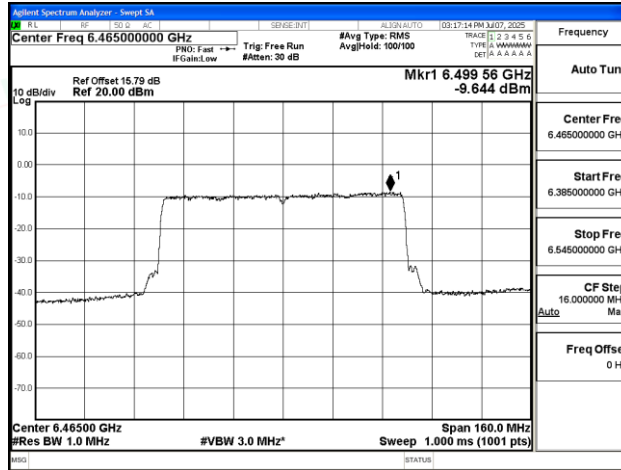
11AX80SISO-Ant2-6465-PASS
