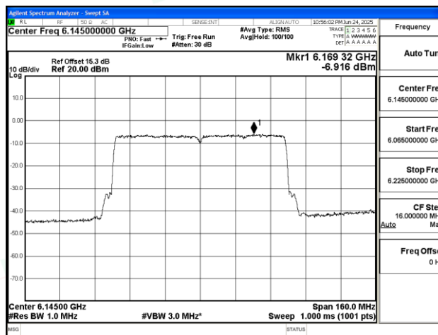
11AX80SISO-Ant1-6145-PASS
