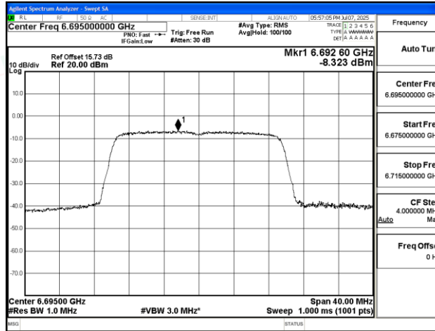
11AX20SISO-Ant1-6695-PASS
