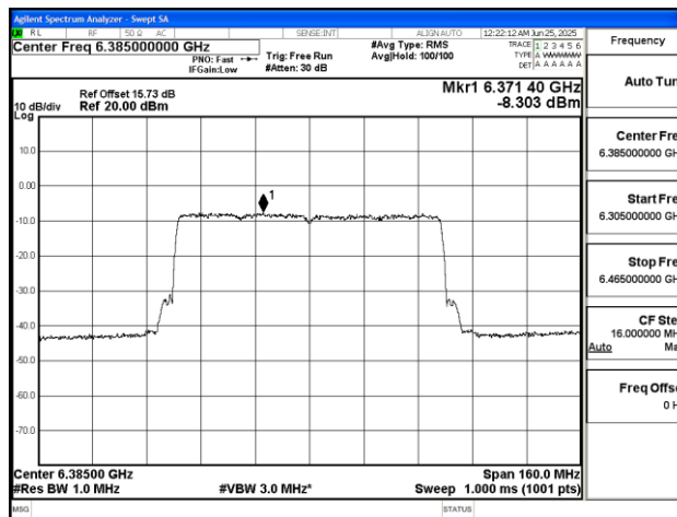
11AX80SISO-Ant2-6385-PASS
