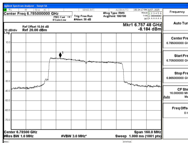
11AX80SISO-Ant1-6785-PASS
