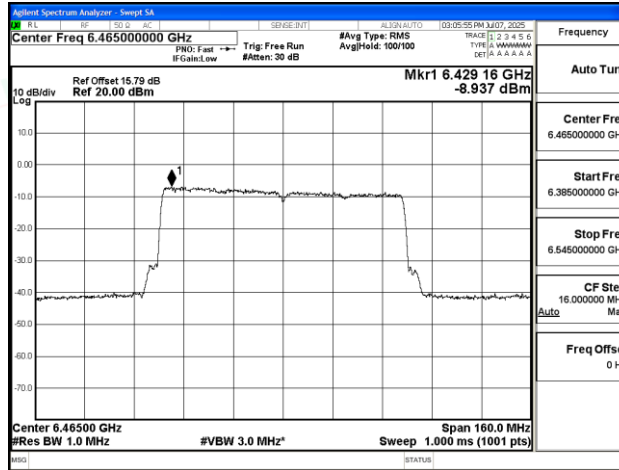
11AX80SISO-Ant1-6465-PASS
