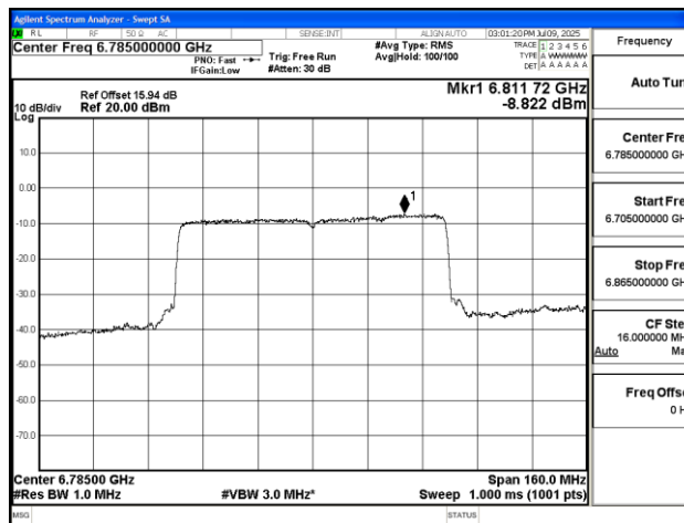
11AX80SISO-Ant2-6785-PASS
