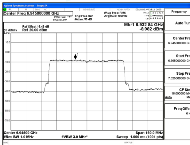
11AX80SISO-Ant1-6945-PASS
