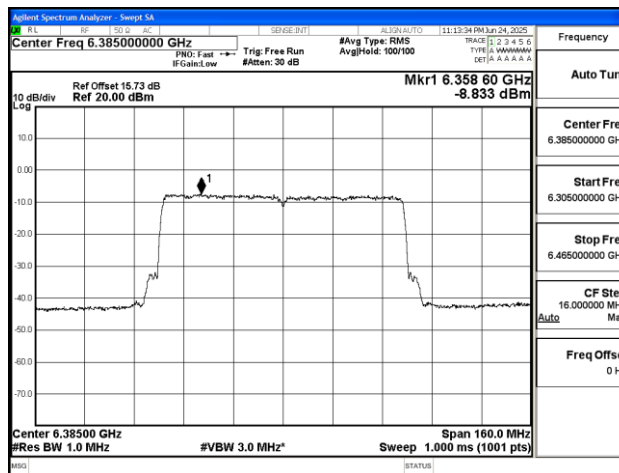
11AX80SISO-Ant1-6385-PASS
