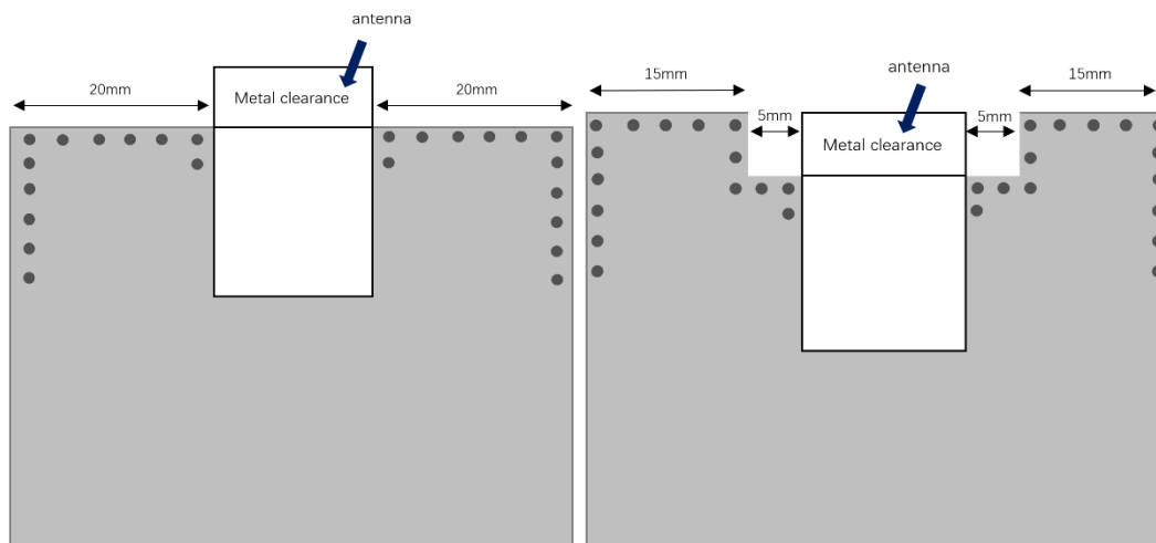
<图 7. PCBA 设计图>
