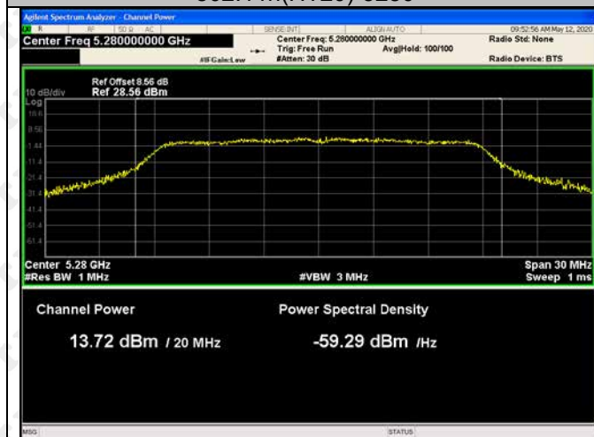
802.11n(HT20)-5280
