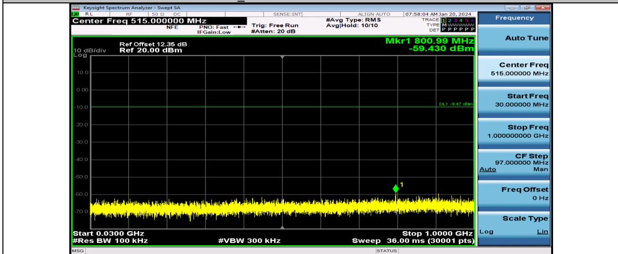
BLE_1M-Ant1-2402-30~1000
