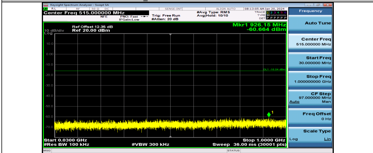
BLE_1M-Ant1-2440-30~1000
