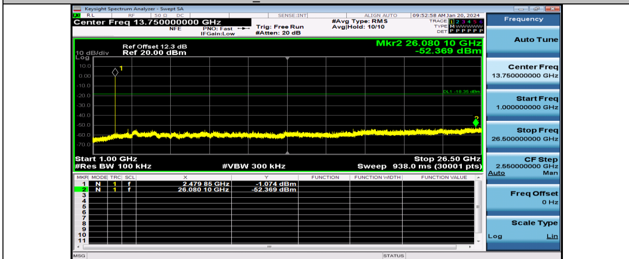
BLE_2M-Ant1-2480-1000~26500
