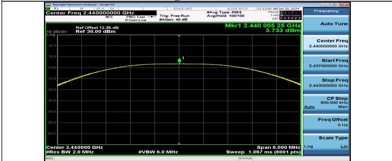
BLE_2M-Ant1-2440
