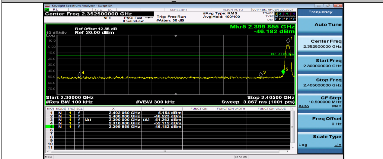
BLE_2M-Ant1-2402
