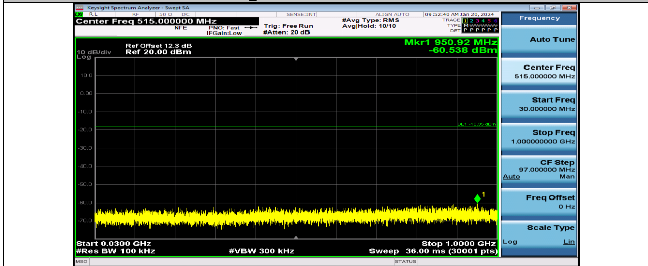
BLE_2M-Ant1-2480-30~1000
