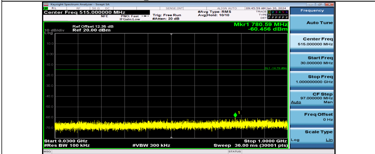
BLE_2M-Ant1-2402-30~1000
