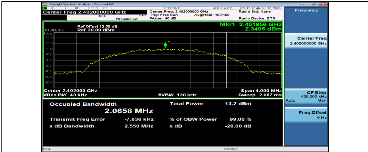
BLE_2M-Ant1-2402
