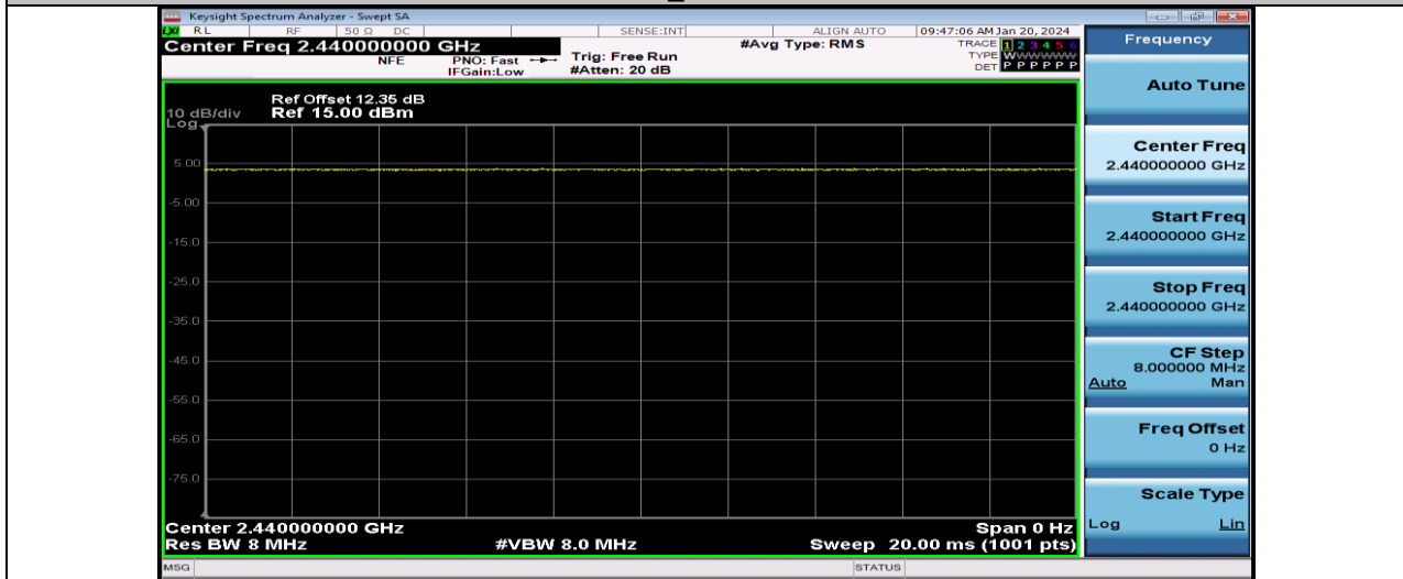
NTNV-BLE_2M-Ant1-2440
