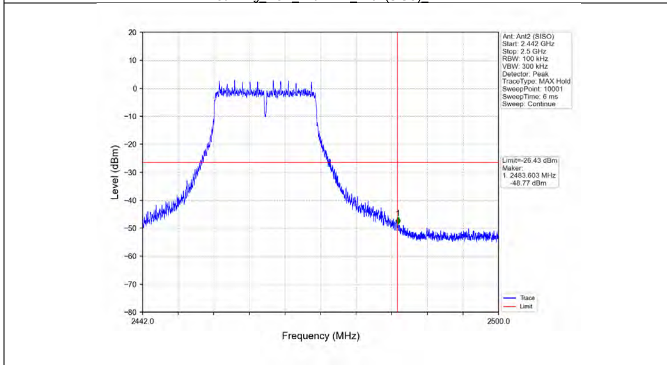
802.11g_HCH_2462MHz_Ant2 (SISO)_NTNV
