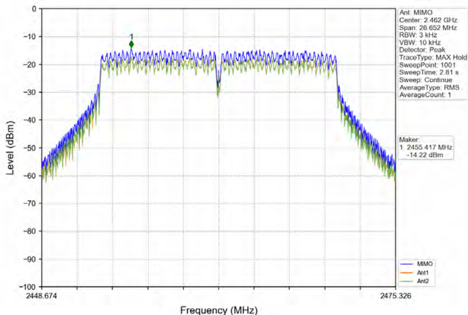
802.11n(HT20) HCH 2462MHz MIMO NTNV
