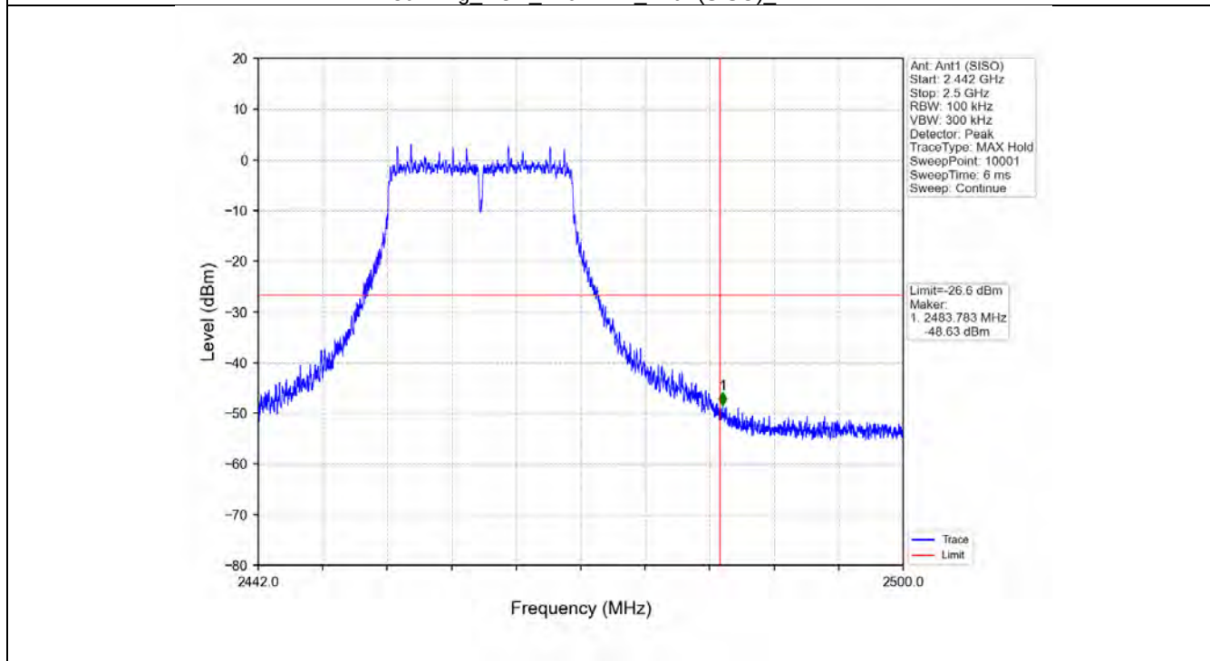
802.11g_HCH_2462MHz_Ant1 (SISO)_NTNV
