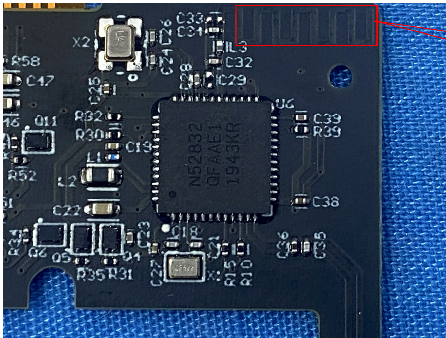
BLE Antenna
