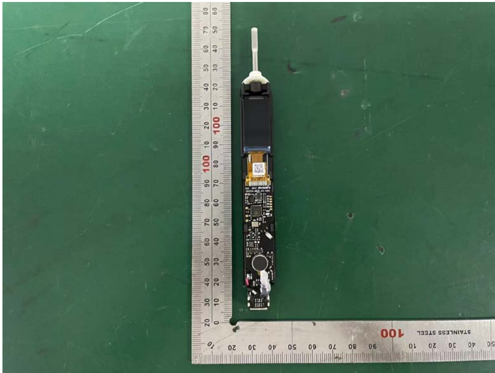
Internal photos M/N: planck mini
