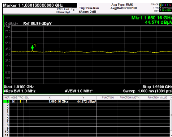
Vertical(1 610-1 990 MHz)
