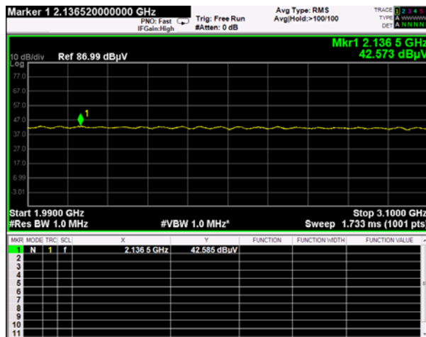
Vertical(1 990-3 100 MHz)
