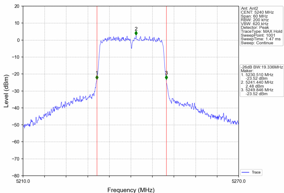
802.11a_HCH_5240MHz_Ant2_NTNV_SISO
