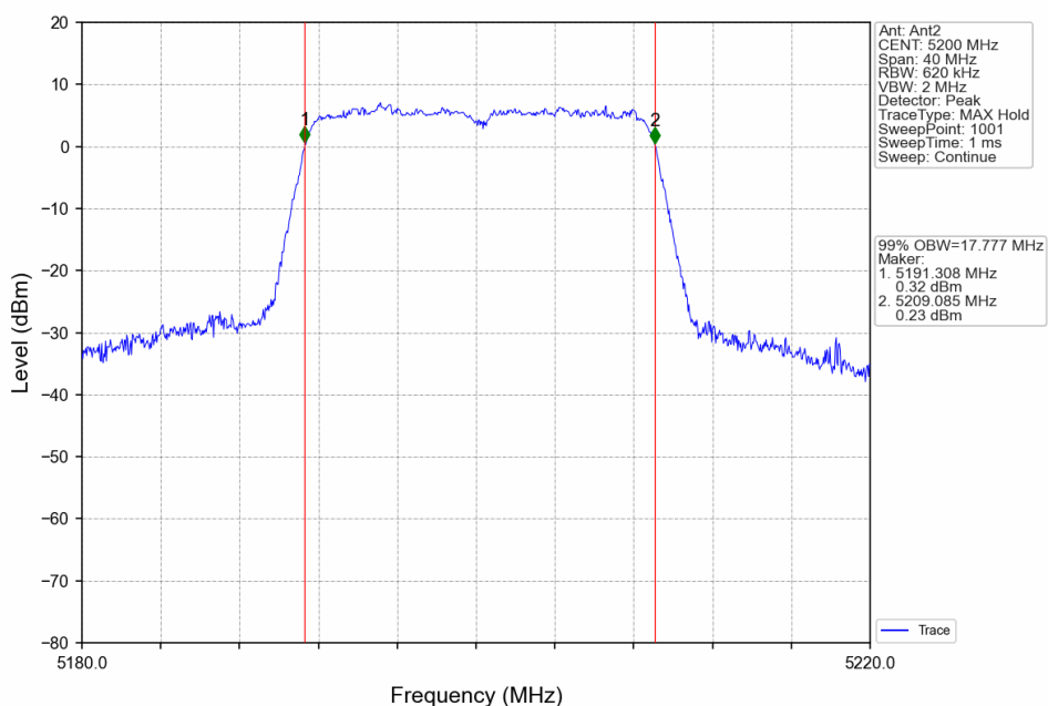
802.11n(HT20)_MCH_5200MHz_Ant2_NTNV_MIMO
