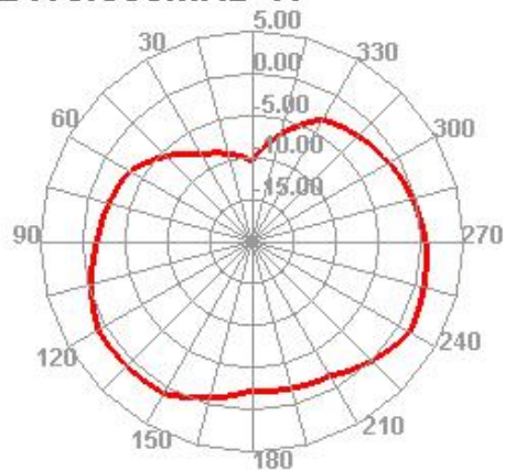
2460.000MHz H
