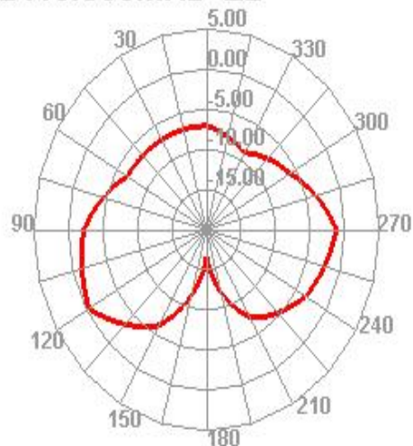
2410.000MHz E2
