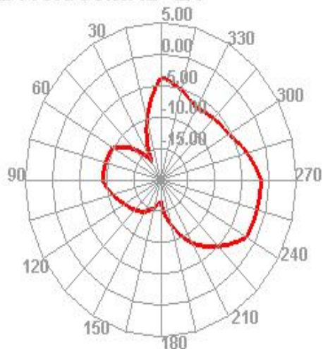
2410.000MHz E1
