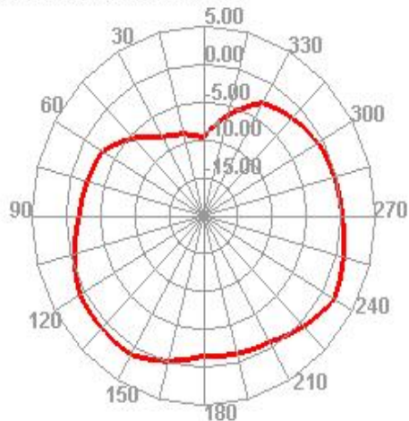
2440.000MHz H
