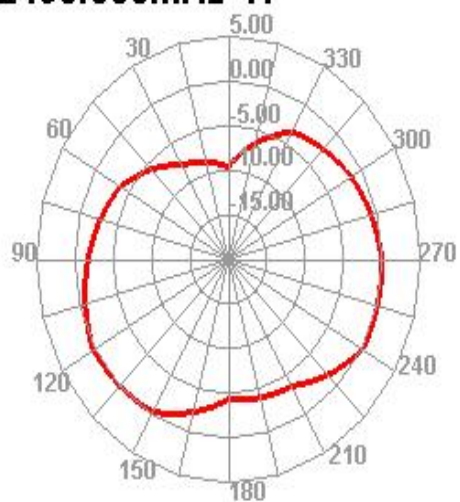
2490.000MHz H
