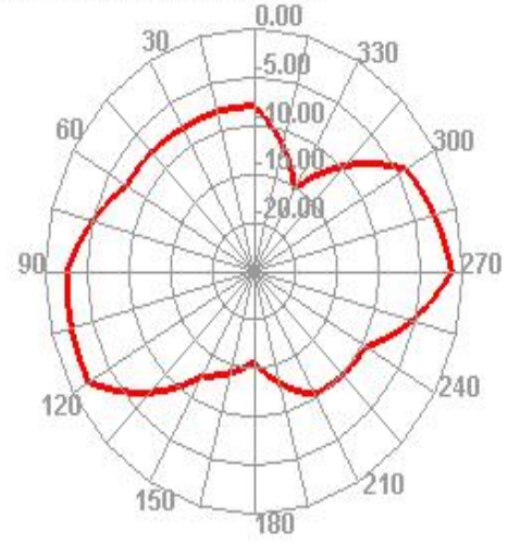
2500.000MHz E2
