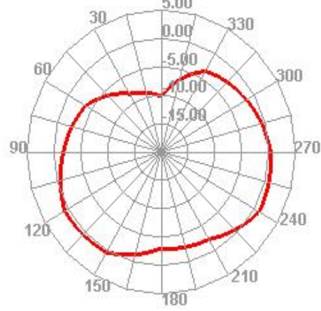
2470.000MHz H
