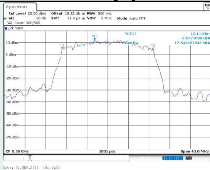
802.11n HT20 MIMO_Ant2_5580MHz
