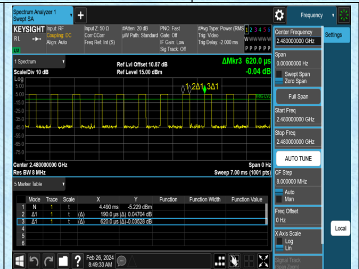
NTNV-BLE_2M-Ant1-2480
