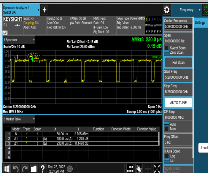
11AC80MIMO_Ant1_5290
