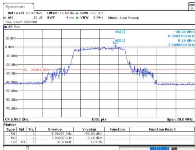
11AX20MIMO_Ant2_6995
