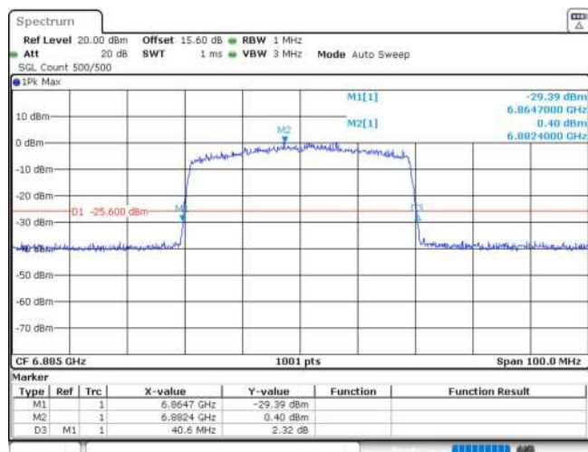
11AX40MIMO_Ant1_6885
