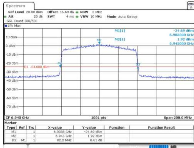
11AX80MIMO_Ant2_6945
