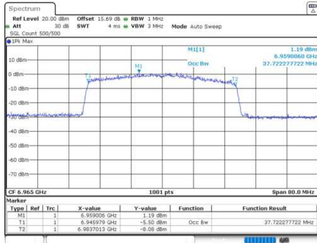
11AX40MIMO_Ant2_6965
