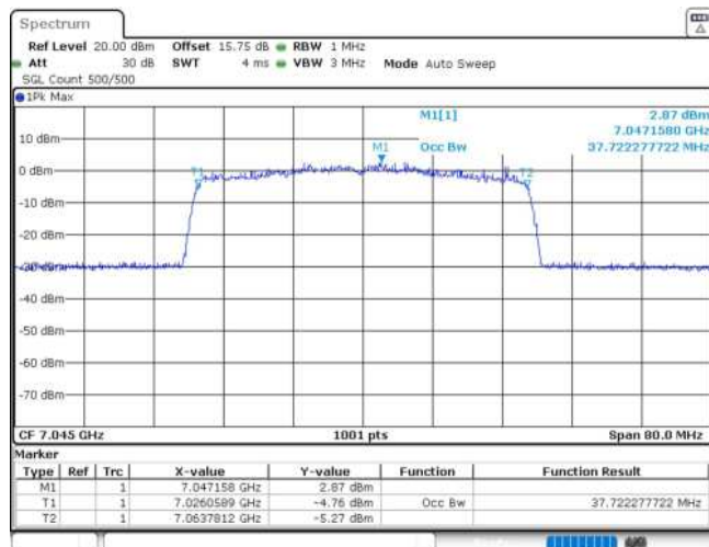
11AX40MIMO_Ant1_7045
