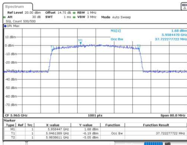
11AX40MIMO_Ant1_5965
