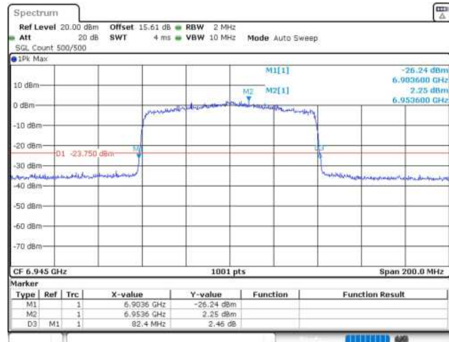
11AX80MIMO_Ant1_6945
