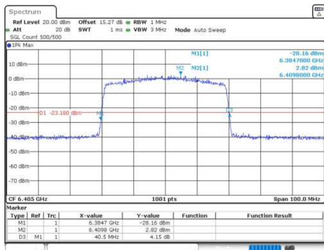
11AX40MIMO_Ant1_6405
