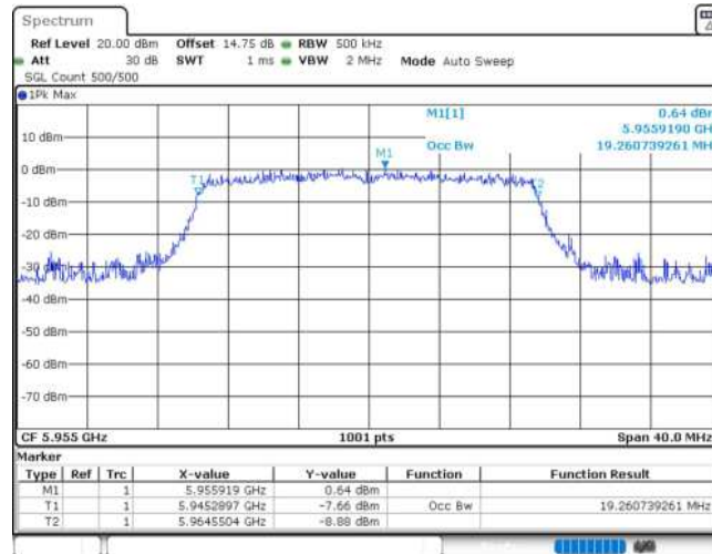
11AX20MIMO_Ant1_5955
