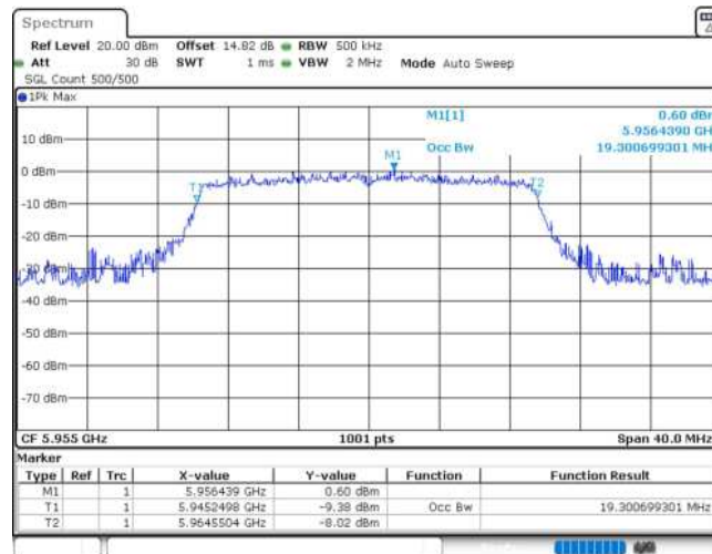
11AX20MIMO_Ant2_5955
