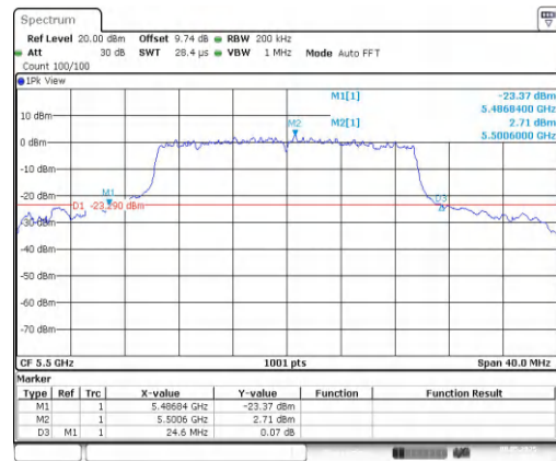
11AX20MIMO-Ant2-5500
