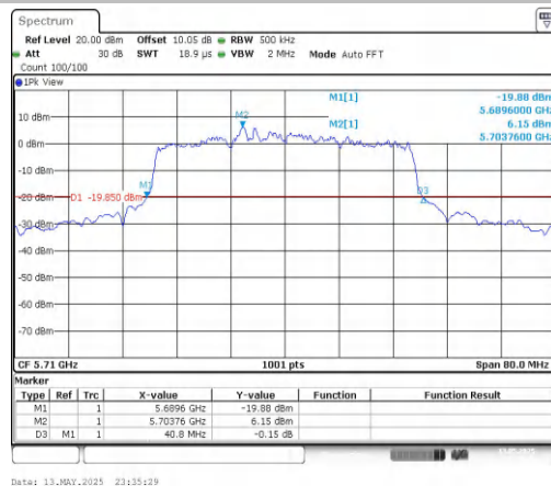
11AX40MIMO-Ant2-5710
