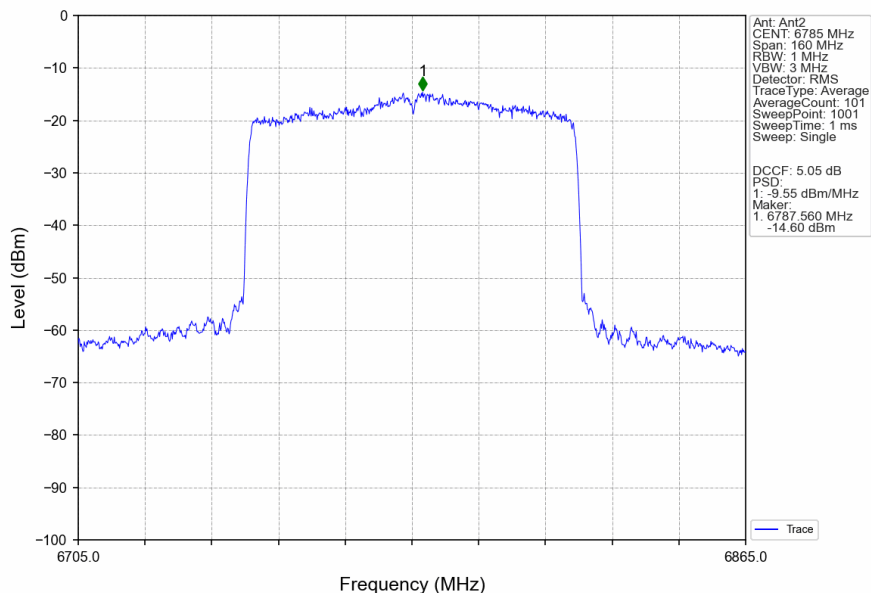
802.11ax(HEW80)_HCH_6785MHz_RU996_Left_Ant2_NTNV
