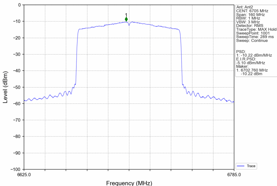
802.11ax(HEW80)_MCH_6705MHz_RU996_Left_Ant2_NTNV
