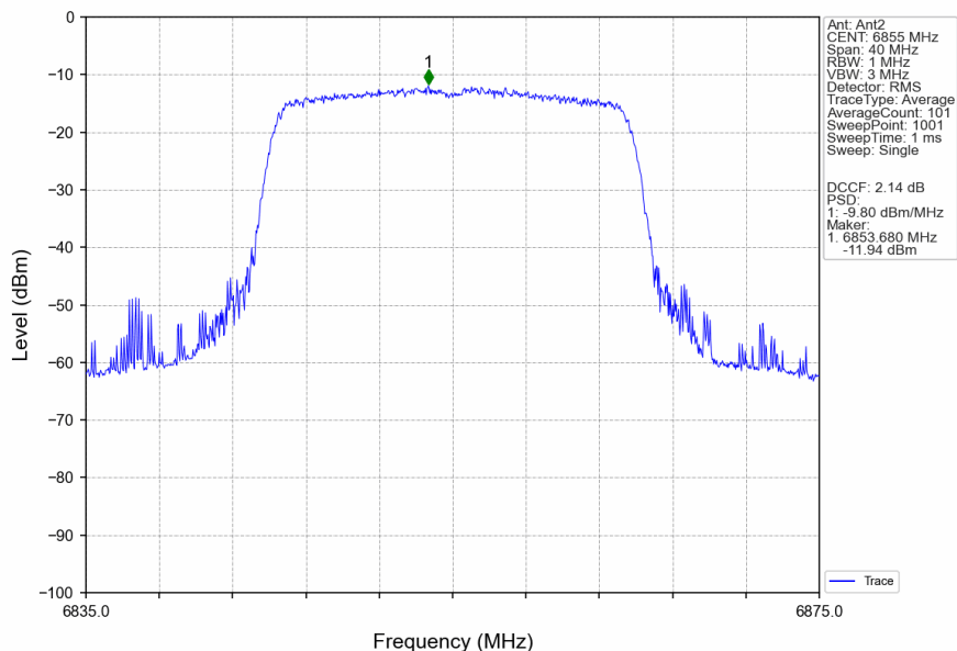
802.11ax(HEW20)_HCH_6855MHz_RU242_Left_Ant2_NTNV
