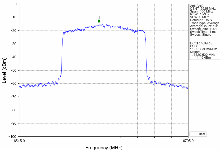
802.11ax(HEW80)_LCH_6625MHz_RU996_Left_Ant2_NTNV
