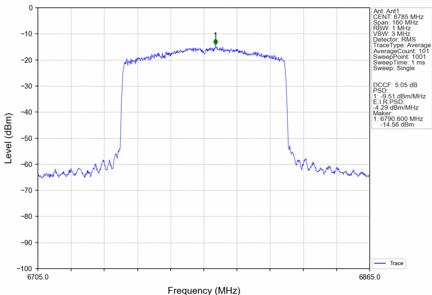
802.11ax(HEW80)_HCH_6785MHz_RU996_Left_Ant1_NTNV
