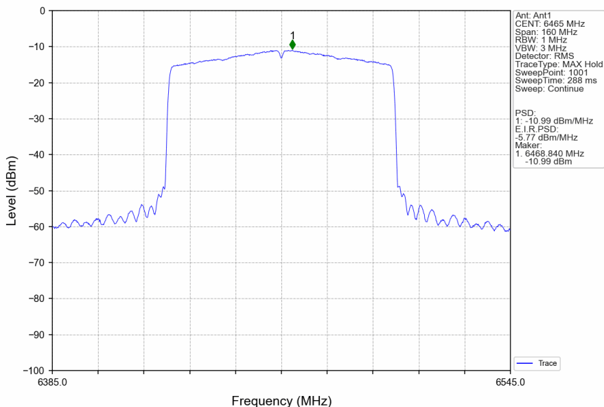
802.11ax(HEW80)_LCH_6465MHz_RU996_Left_Ant1_NTNV
