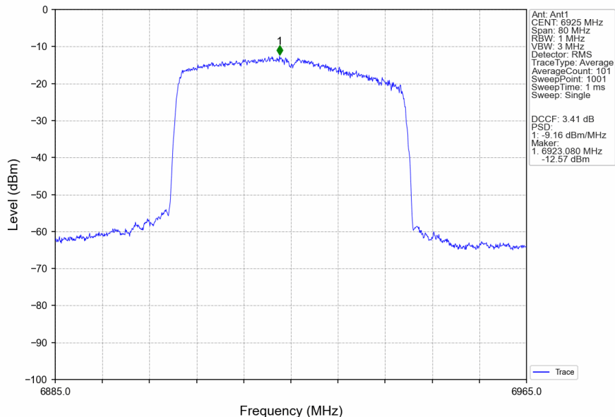
802.11ax(HEW40)_LCH_6925MHz_RU484_Left_Ant1_NTNV
