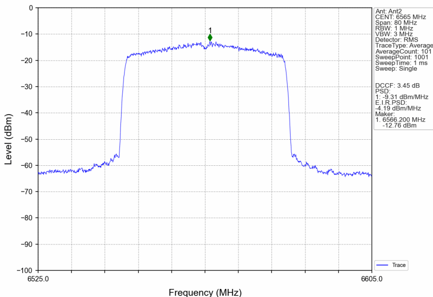
802.11ax(HEW40)_LCH_6565MHz_RU484_Left_Ant2_NTNV
