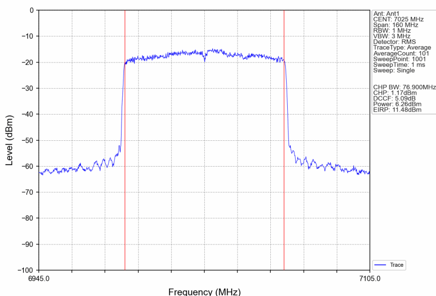
802.11ax(HEW80)_HCH_7025MHz_RU996_Left_Ant1_NTNV
