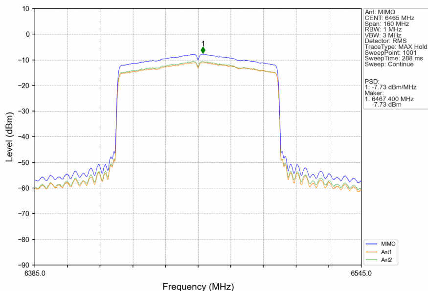
802.11ax(HEW80)_LCH_6465MHz_RU996_Left_MIMO_NTNV
