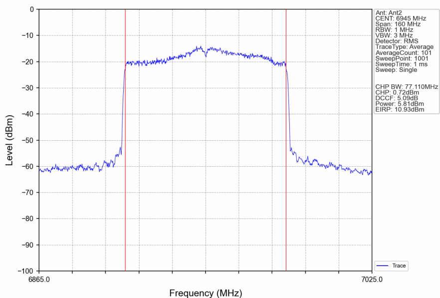
802.11ax(HEW80)_LCH_6945MHz_RU996_Left_Ant2_NTNV
