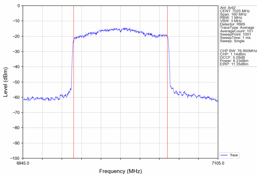
802.11ax(HEW80)_HCH_7025MHz_RU996_Left_Ant2_NTNV
