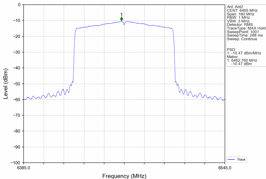
802.11ax(HEW80)_LCH_6465MHz_RU996_Left_MIMO_NTNV
