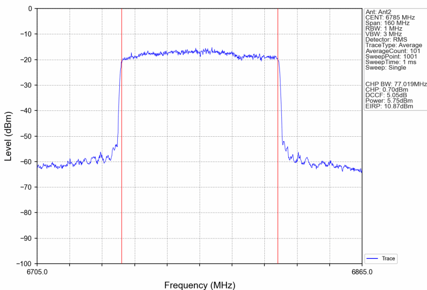
802.11ax(HEW80)_HCH_6785MHz_RU996_Left_Ant2_NTNV
