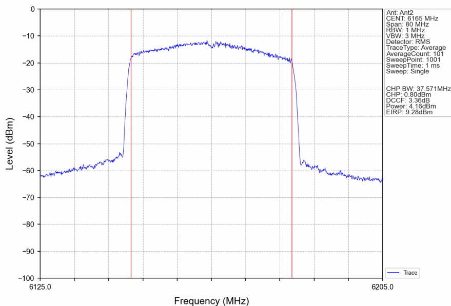
802.11ax(HEW40)_MCH_6165MHz_RU484_Left_Ant2_NTNV
