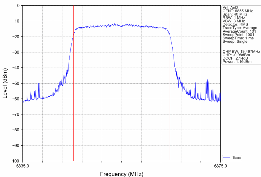
802.11ax(HEW20)_HCH_6855MHz_RU242_Left_Ant2_NTNV
