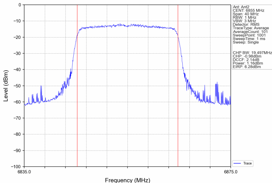
802.11ax(HEW20)_HCH_6855MHz_RU242_Left_Ant2_NTNV
