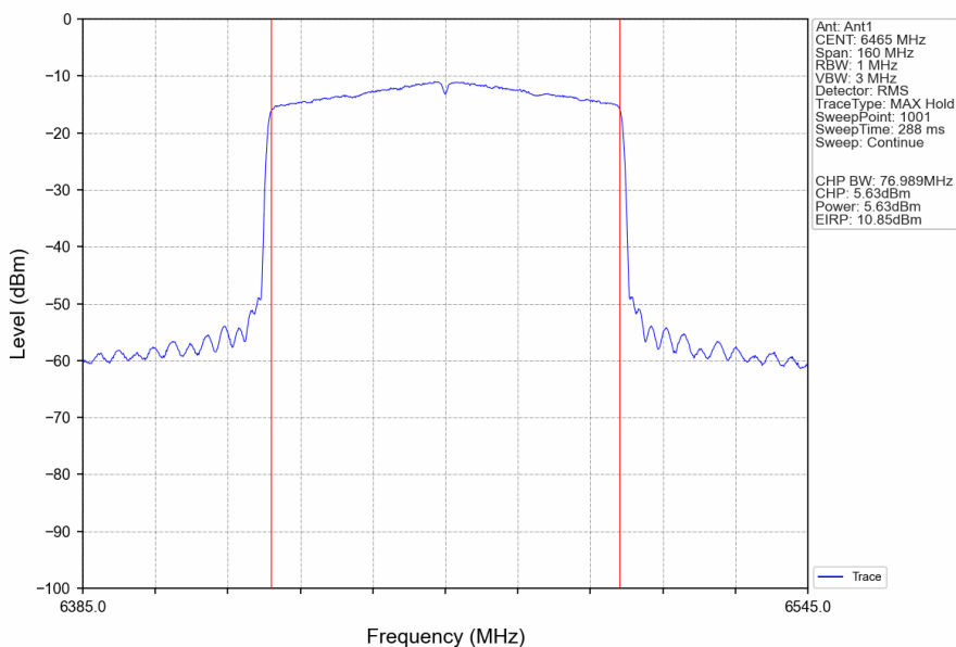
802.11ax(HEW80)_LCH_6465MHz_RU996_Left_Ant1_NTNV
