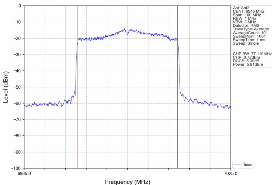
802.11ax(HEW80)_LCH_6945MHz_RU996_Left_Ant2_NTNV
