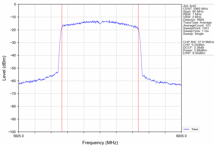
802.11ax(HEW40)_LCH_5965MHz_RU484_Left_Ant2_NTNV
