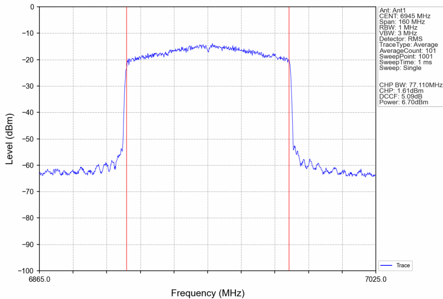
802.11ax(HEW80)_LCH_6945MHz_RU996_Left_Ant1_NTNV
