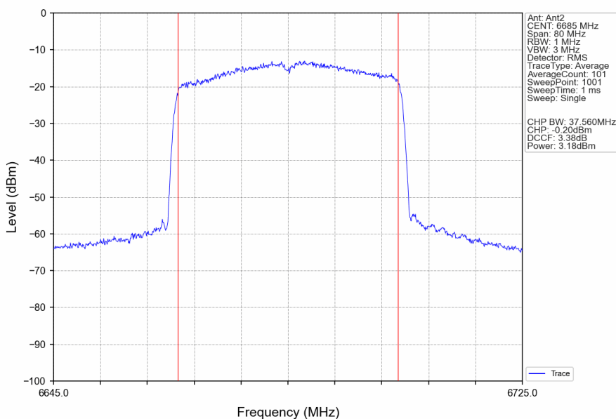
802.11ax(HEW40)_MCH_6685MHz_RU484_Left_Ant2_NTNV
