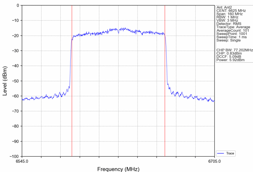
802.11ax(HEW80)_LCH_6625MHz_RU996_Left_Ant2_NTNV
