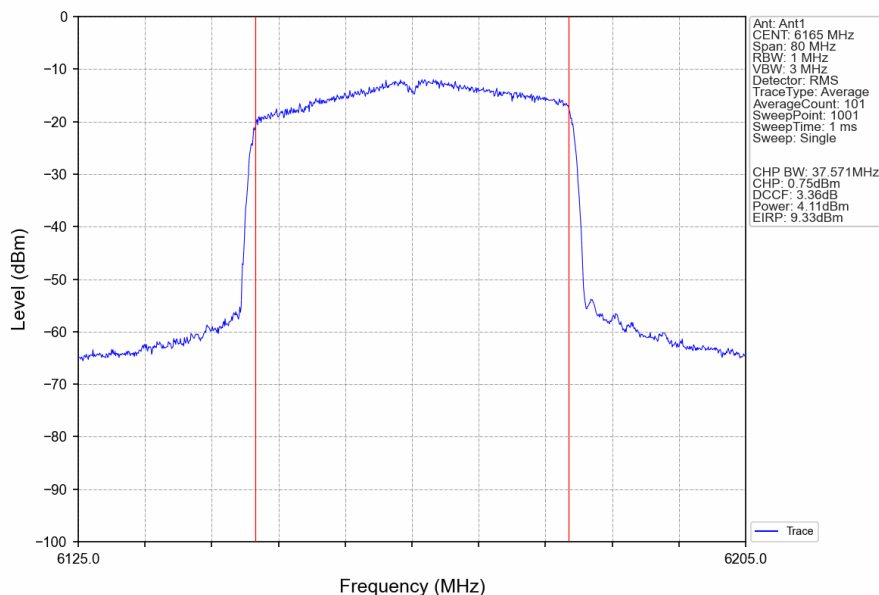
802.11ax(HEW40)_MCH_6165MHz_RU484_Left_Ant1_NTNV
