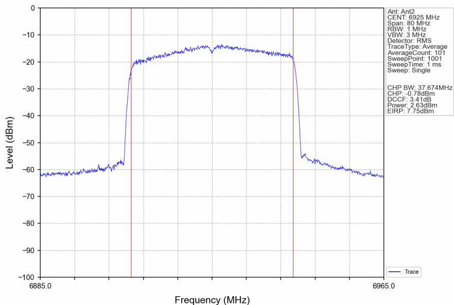
802.11ax(HEW40)_LCH_6925MHz_RU484_Left_Ant2_NTNV
