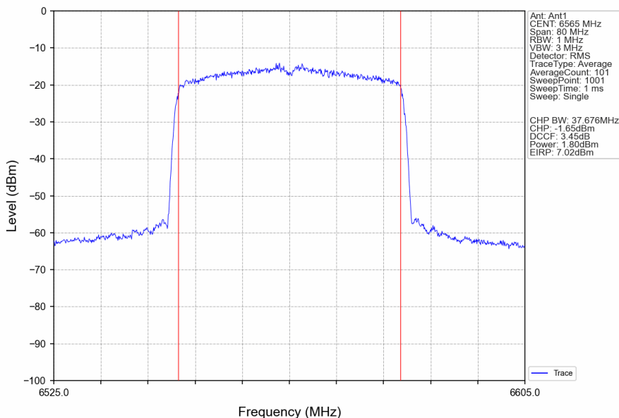
802.11ax(HEW40)_LCH_6565MHz_RU484_Left_Ant1_NTNV
