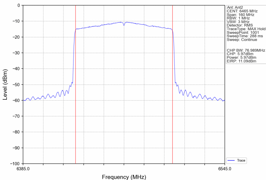
802.11ax(HEW80)_LCH_6465MHz_RU996_Left_Ant2_NTNV
