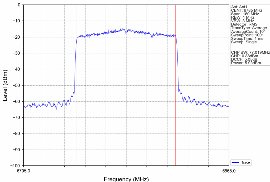
802.11ax(HEW80)_HCH_6785MHz_RU996_Left_Ant1_NTNV
