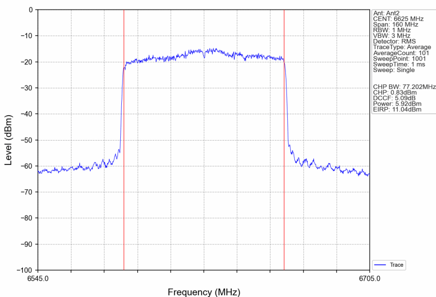
802.11ax(HEW80)_LCH_6625MHz_RU996_Left_Ant2_NTNV
