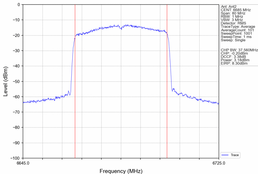
802.11ax(HEW40)_MCH_6685MHz_RU484_Left_Ant2_NTNV
