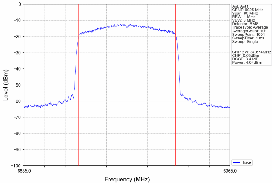
802.11ax(HEW40)_LCH_6925MHz_RU484_Left_Ant1_NTNV
