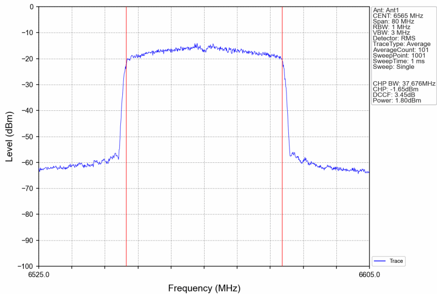
802.11ax(HEW40)_LCH_6565MHz_RU484_Left_Ant1_NTNV
