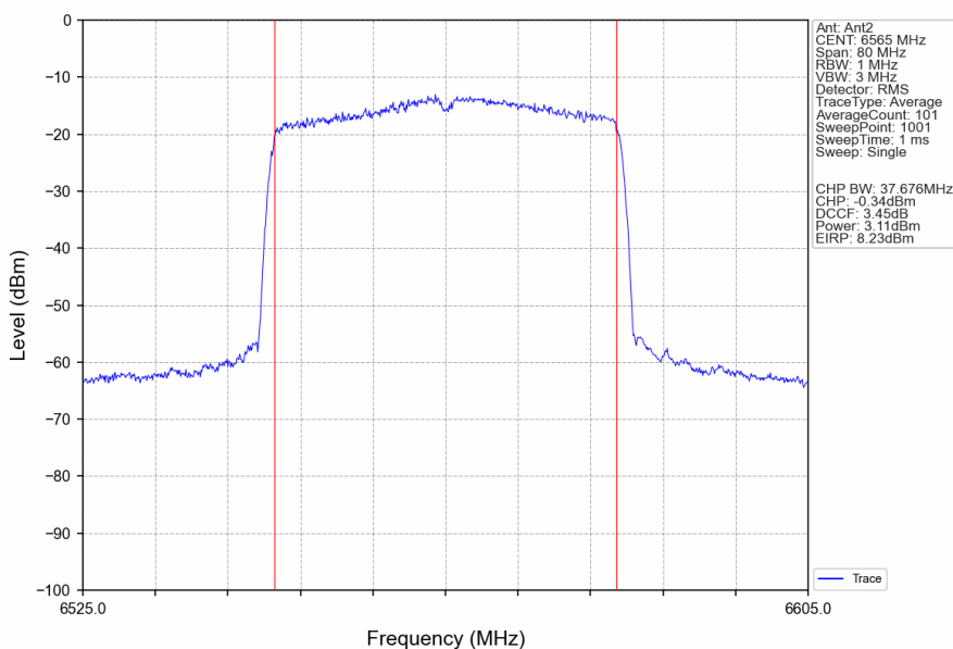
802.11ax(HEW40)_LCH_6565MHz_RU484_Left_Ant2_NTNV
