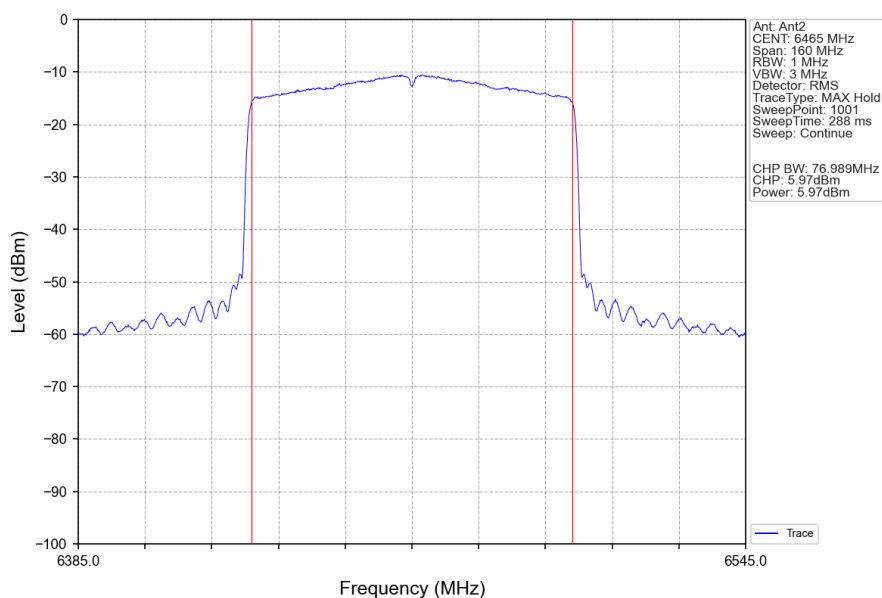
802.11ax(HEW80)_LCH_6465MHz_RU996_Left_Ant2_NTNV
