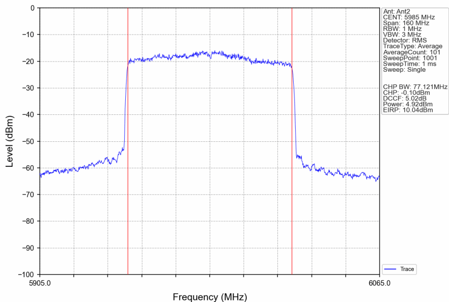
802.11ax(HEW80)_LCH_5985MHz_RU996_Left_Ant2_NTNV
