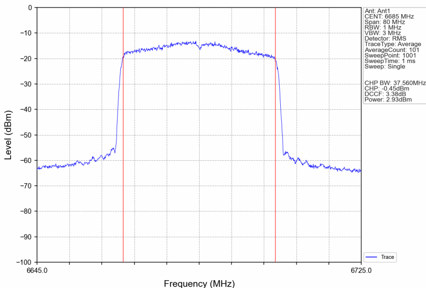
802.11ax(HEW40)_MCH_6685MHz_RU484_Left_Ant1_NTNV
