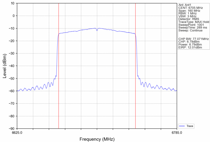
802.11ax(HEW80)_MCH_6705MHz_RU996_Left_Ant1_NTNV
