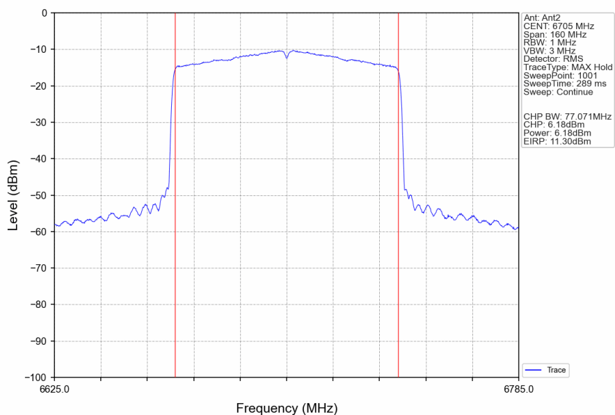
802.11ax(HEW80)_MCH_6705MHz_RU996_Left_Ant2_NTNV
