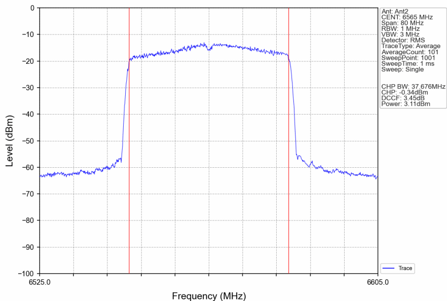
802.11ax(HEW40)_LCH_6565MHz_RU484_Left_Ant2_NTNV
