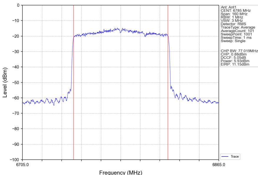
802.11ax(HEW80)_HCH_6785MHz_RU996_Left_Ant1_NTNV
