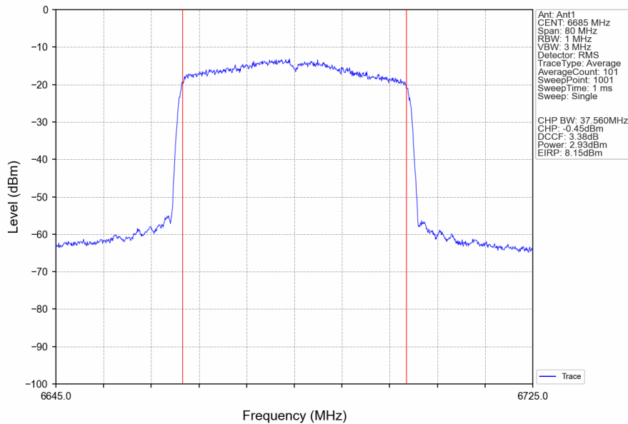
802.11ax(HEW40)_MCH_6685MHz_RU484_Left_Ant1_NTNV
