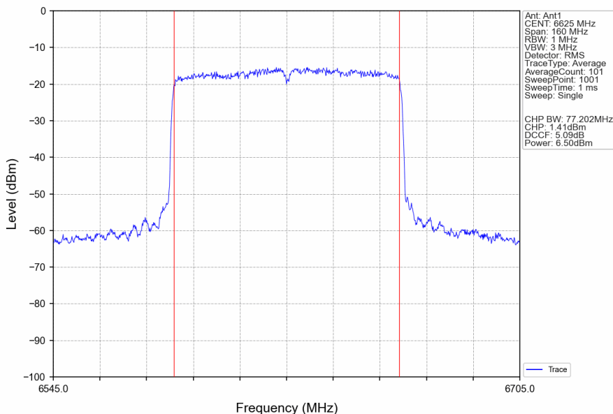
802.11ax(HEW80)_LCH_6625MHz_RU996_Left_Ant1_NTNV
