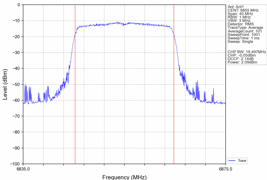
802.11ax(HEW20)_HCH_6855MHz_RU242_Left_Ant1_NTNV
