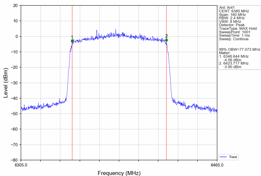
802.11ax(HEW80)_HCH_6385MHz_RU996_Left_Ant1_NTNV
