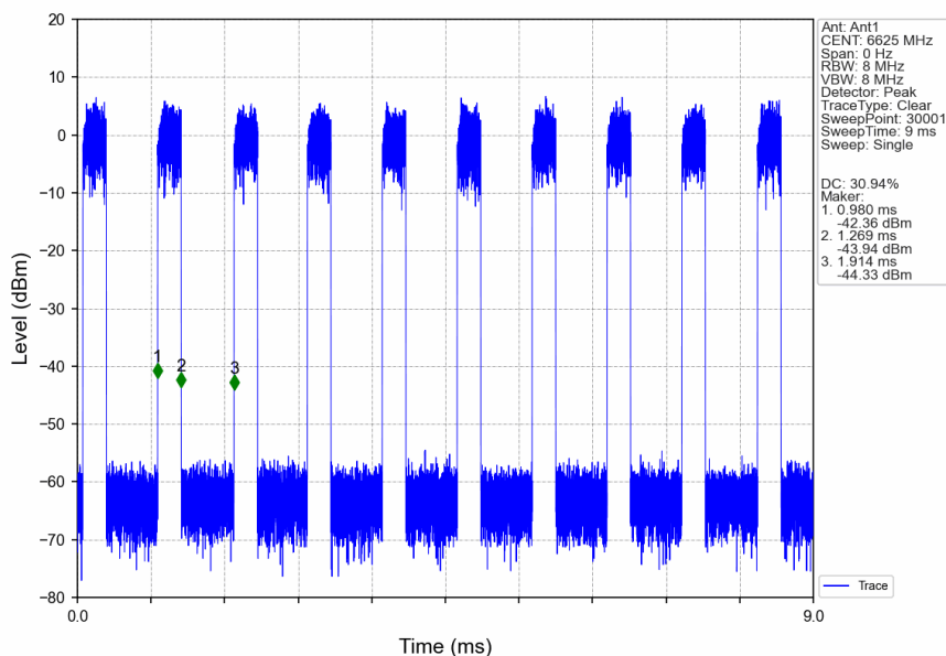
802.11ax(HEW80)_LCH_6625MHz_RU996_Left_Ant1_NTNV
