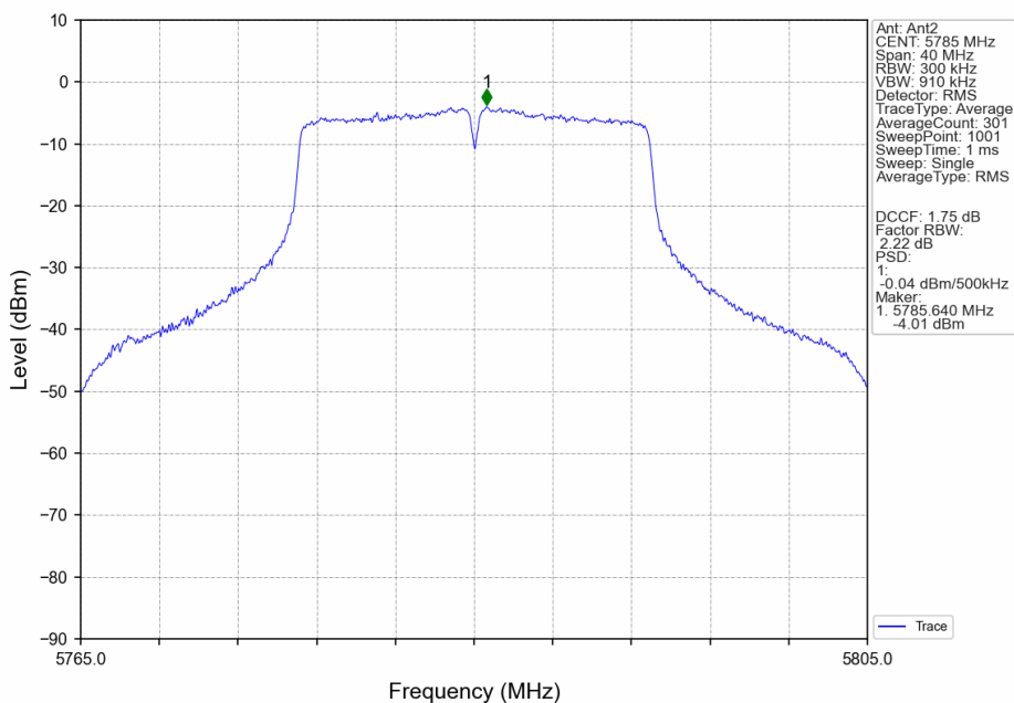
802.11n(HT20)_MCH_5785MHz_MIMO_NTNV
