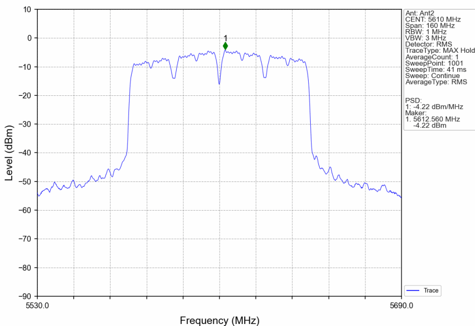
802.11ax(HEW80)_HCH_5610MHz_SU_/_MIMO_NTNV
