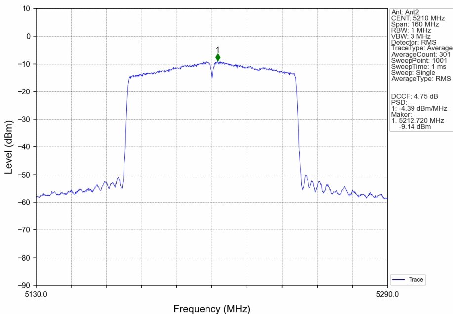
802.11ac(VHT80)_MCH_5210MHz_Ant2_NTNV
