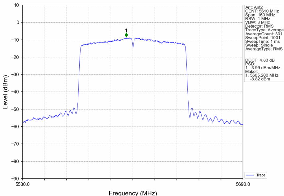
802.11ac(VHT80)_HCH_5610MHz_MIMO_NTNV
