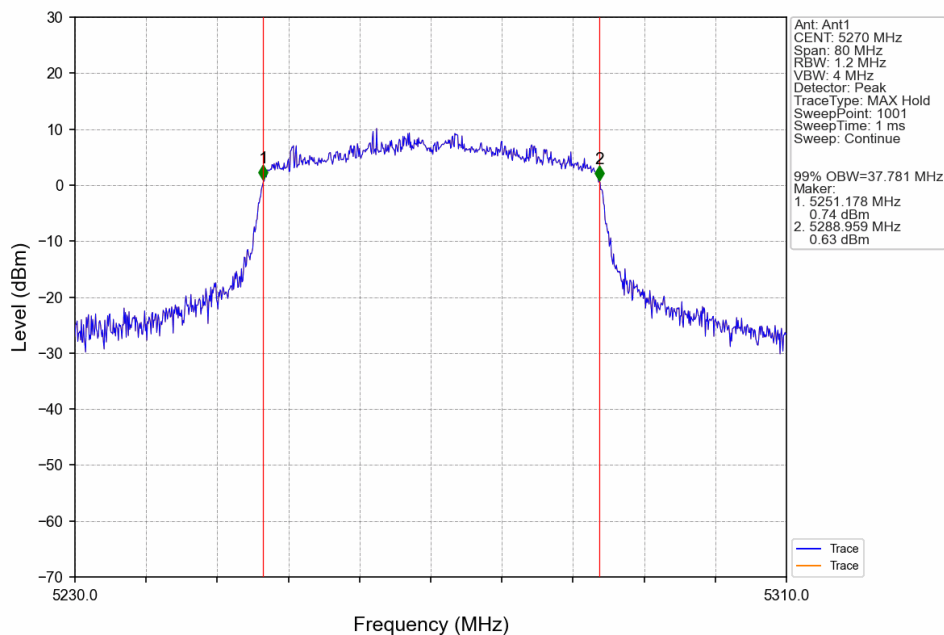
802.11ax(HEW40)_LCH_5270MHz_SU_ / _Ant1_NTNV
