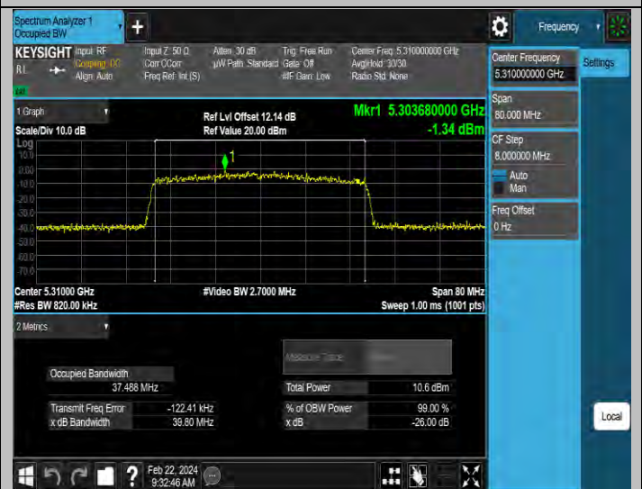
11AX40MIMO-Ant2-5310
