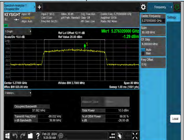
11AX40MIMO-Ant2-5270
