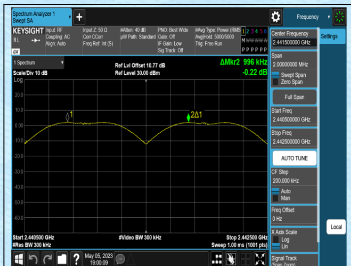
DH5-Ant1-Hop
