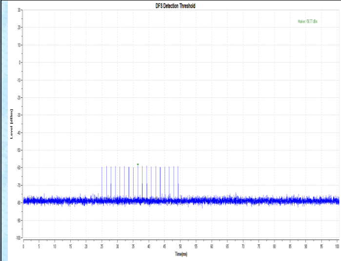
11AC80SISO-5290-Type0-PASS
