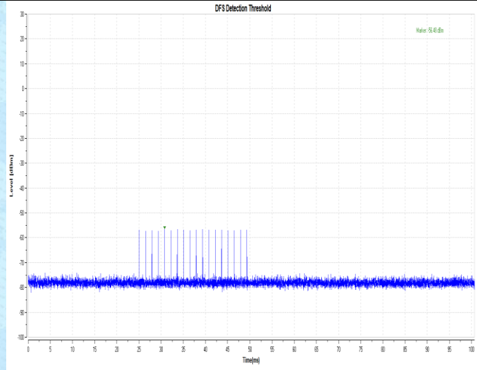
11AC80SISO-5530-Type0-PASS
