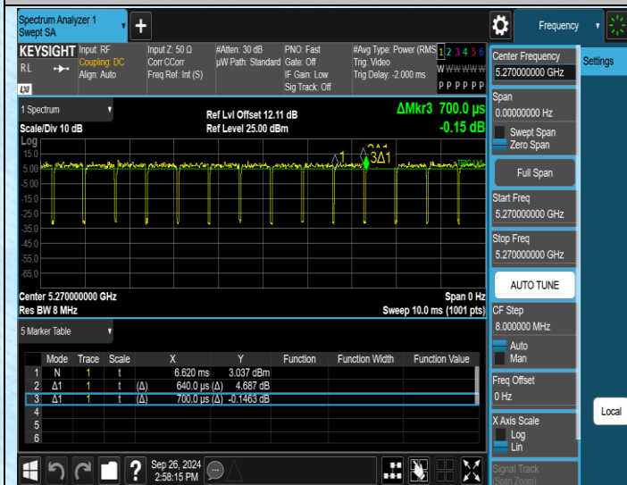
NTNV-11N40MIMO-Ant1-5270
