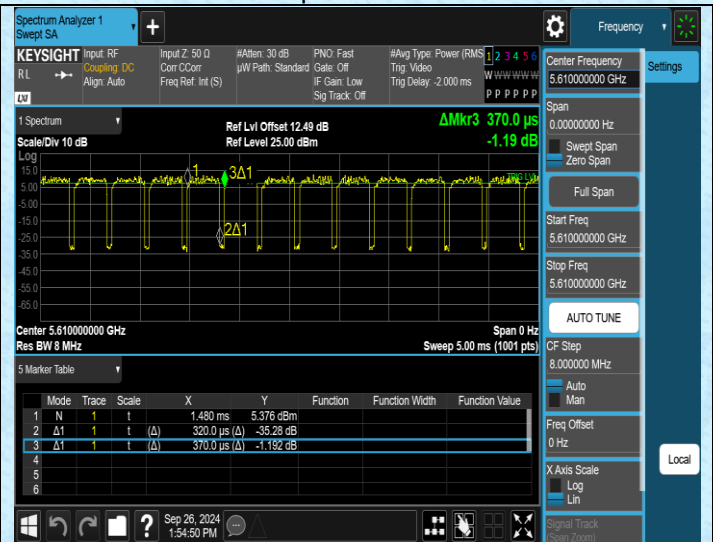
NTNV-11AC80SISO-Ant2-5610
