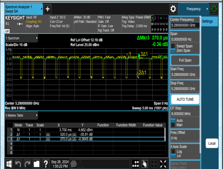
NTNV-11AC80SISO-Ant2-5290
