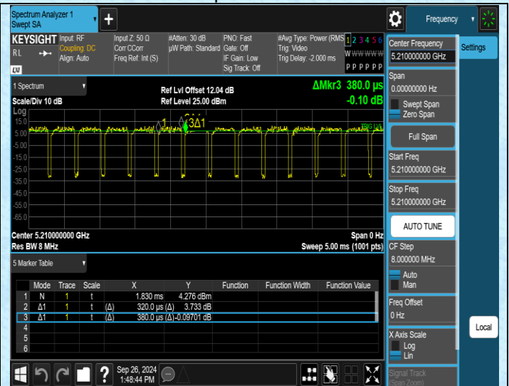
NTNV-11AC80SISO-Ant2-5210
