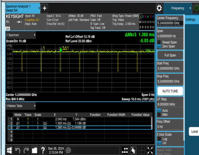
NTNV-11N20MIMO-Ant1-5240
