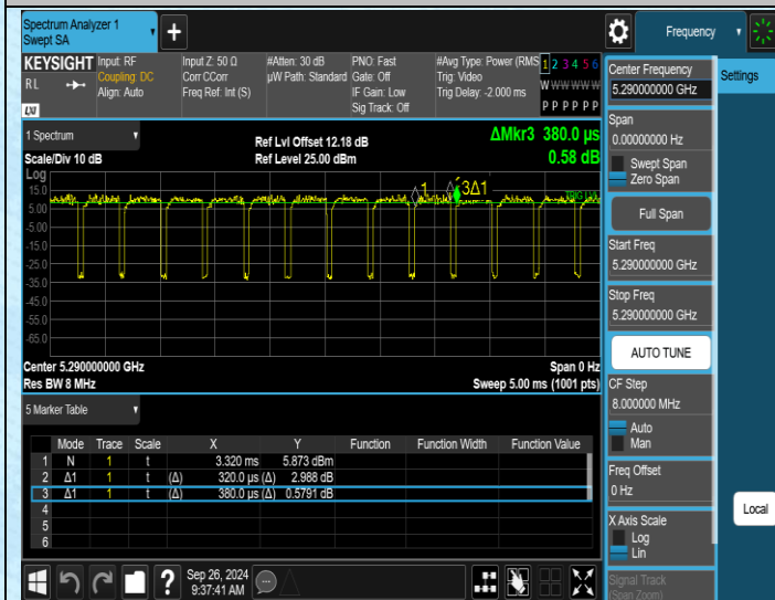
NTNV-11AC80SISO-Ant1-5290
