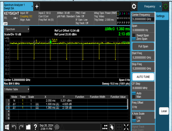
NTNV-11N20MIMO-Ant2-5200
