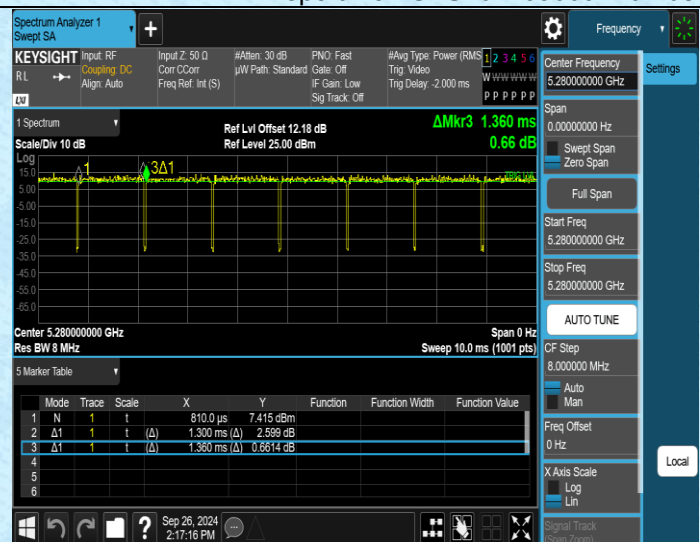
NTNV-11N20MIMO-Ant2-5280
