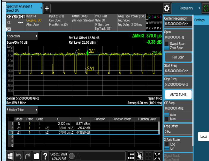
NTNV-11AC80SISO-Ant1-5530
