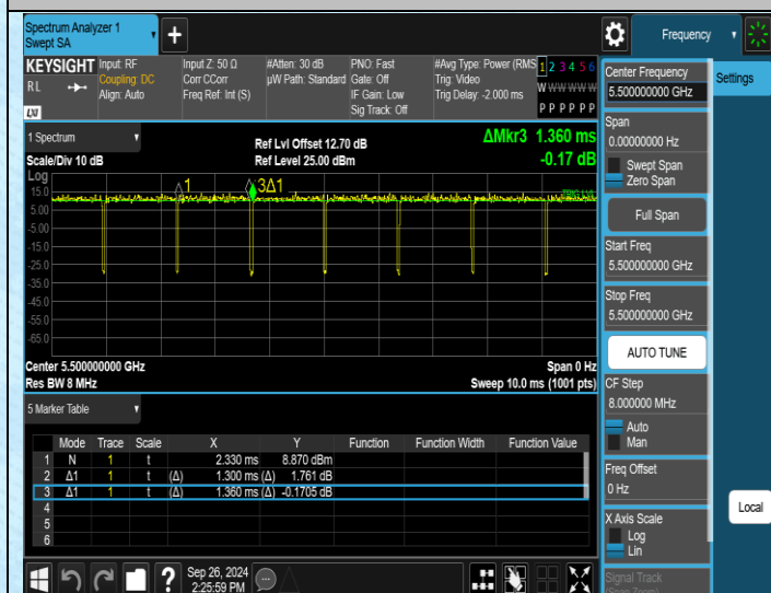
NTNV-11N20MIMO-Ant1-5500
