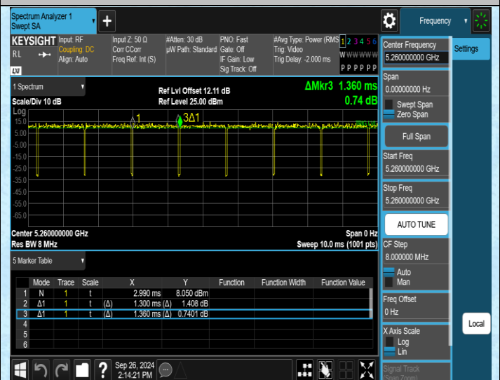
NTNV-11N20MIMO-Ant2-5260
