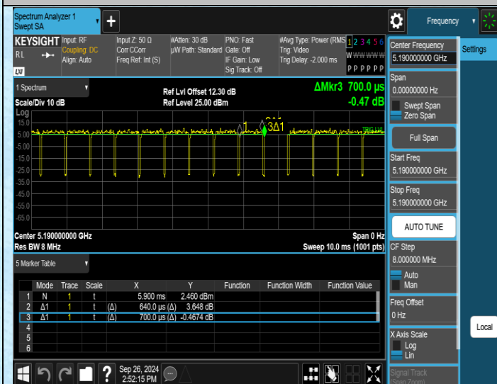
NTNV-11N40MIMO-Ant1-5190
