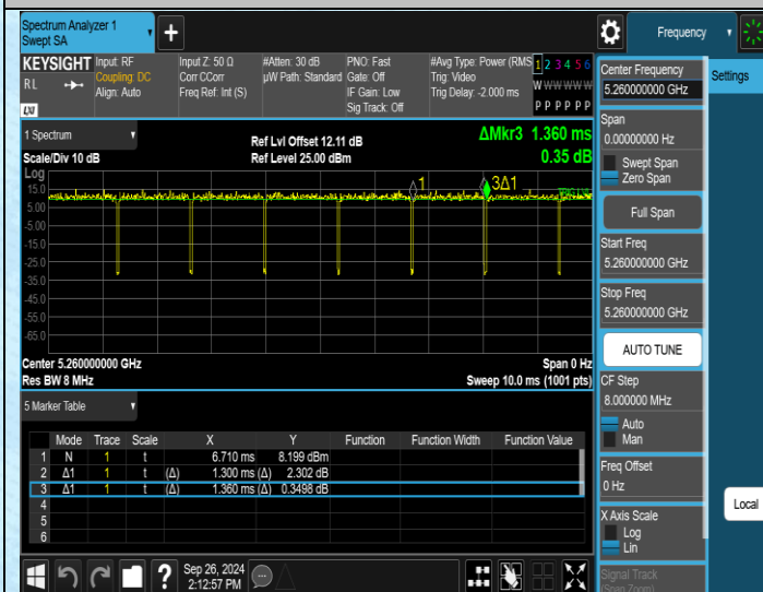
NTNV-11N20MIMO-Ant1-5260
