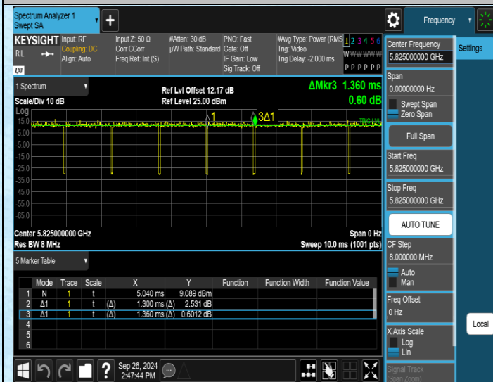
NTNV-11N20MIMO-Ant1-5825
