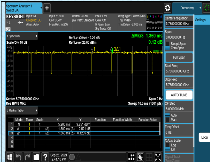
NTNV-11N20MIMO-Ant1-5785
