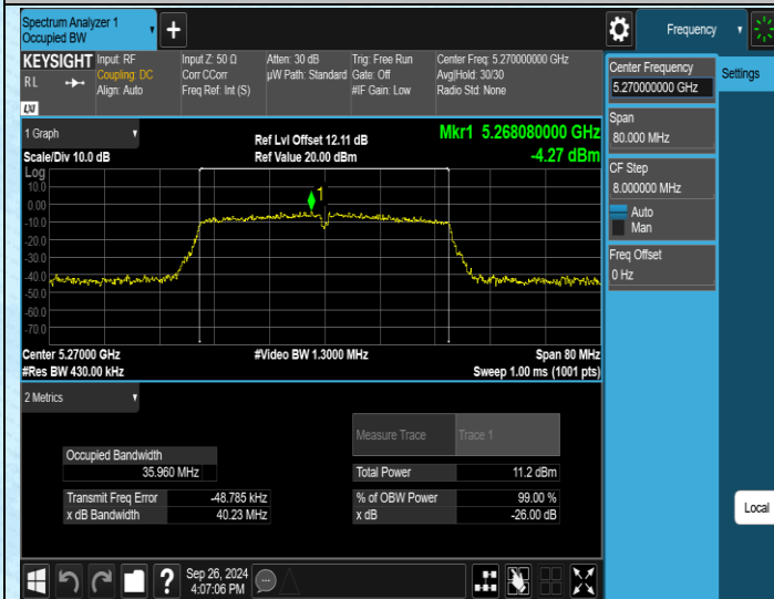
11AC40MIMO-Ant1-5270
