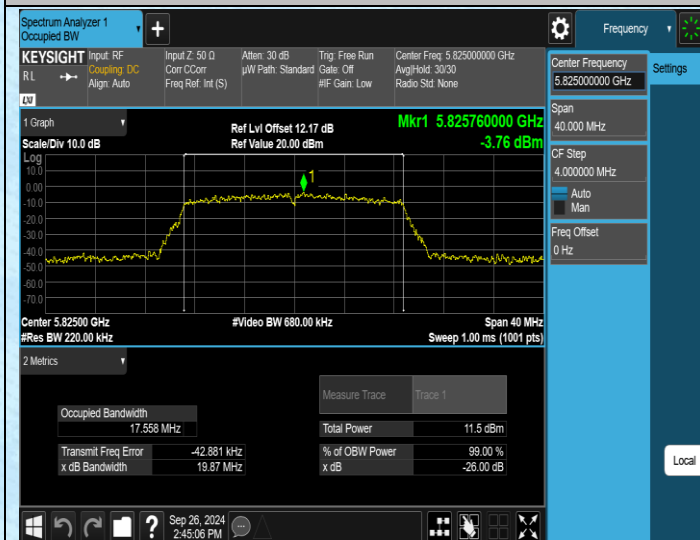
11N20MIMO-Ant1-5825
