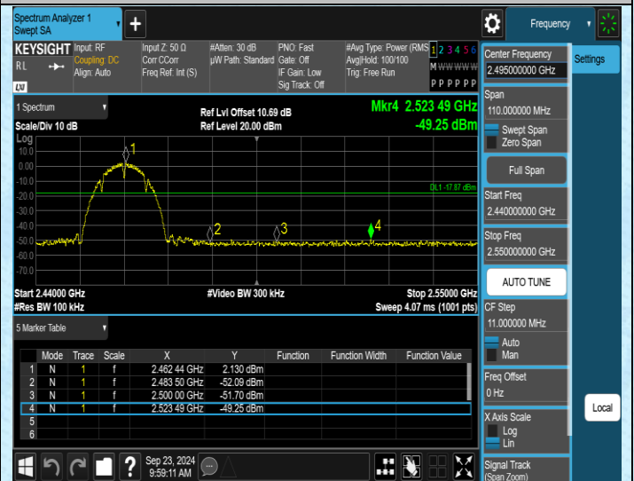
11B-Ant2-2462-PASS
