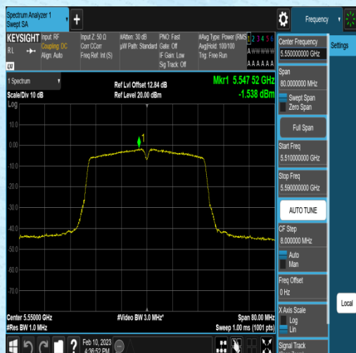
11N40MIMO-Ant1-5550--1.80-0.26-0.00-0.00
