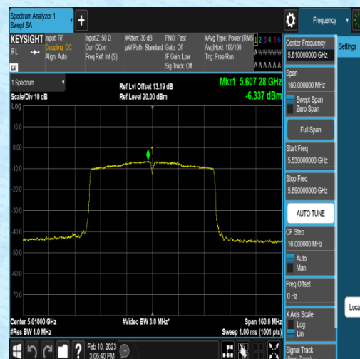
11AC80SISO-Ant2-5610--6.84-0.50-0.00-0.00
