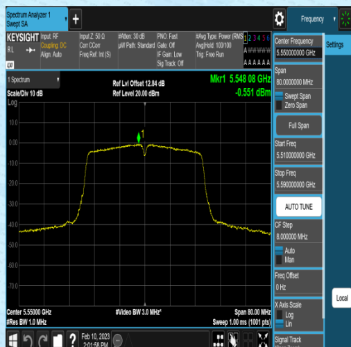
11N40SISO-Ant2-5550--0.81-0.26-0.00-0.00
