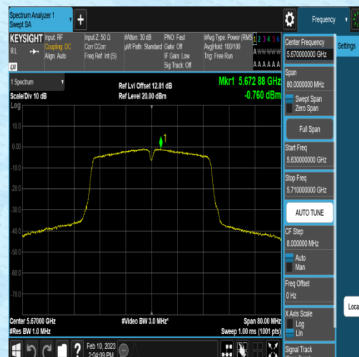
11N40SISO-Ant2-5670--1.02-0.26-0.00-0.00
