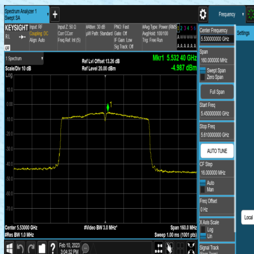
11AC80SISO-Ant2-5530--5.49-0.50-0.00-0.00
