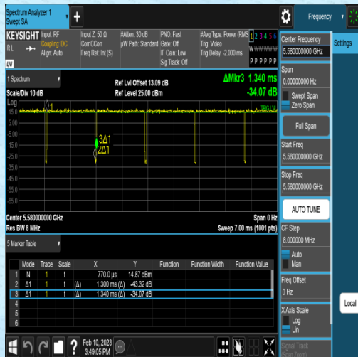
NTNV-11N20MIMO-Ant1-5580-1.30-1.34
