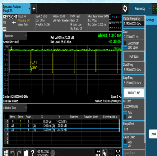
NTNV-11N20MIMO-Ant1-5280-1.30-1.34
