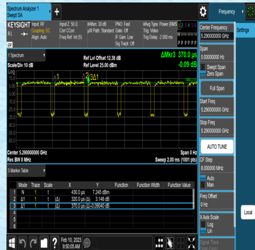
NTNV-11AC80SISO-Ant1-5290-0.32-0.37
