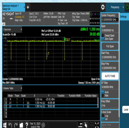
NTNV-11N20MIMO-Ant1-5320-1.30-1.35
