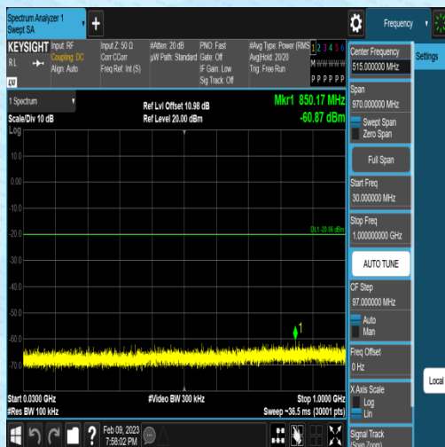
11G-Ant2-2412-30~1000--0.06
