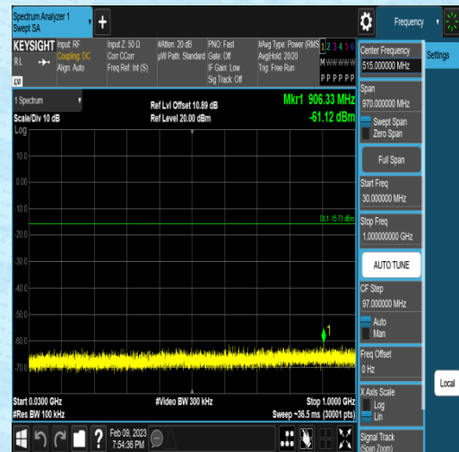
11B-Ant2-2462-30~1000-4.27
