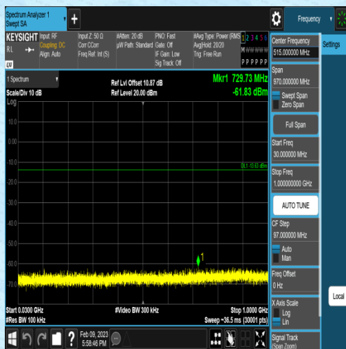
BLE_2M-Ant1-2402-30~1000-6.37
