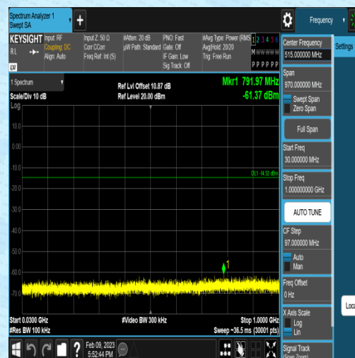
BLE_1M-Ant1-2402-30~1000-5.48
