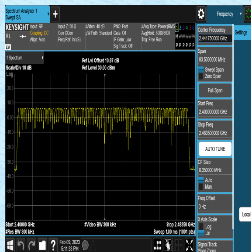
DH5-Ant1-Hop
