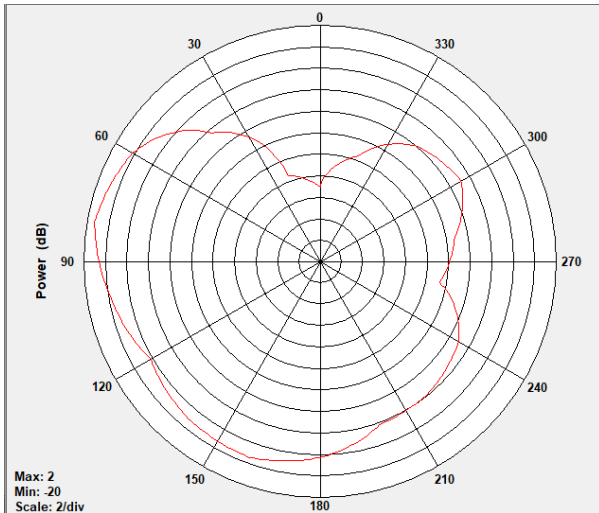
XY-PLANE, f=2403\text{MHz}
