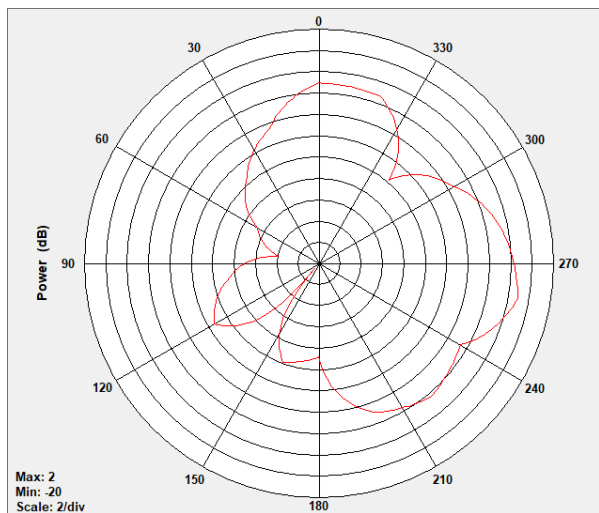
ZX-PLANE, f=2403\text{MHz}
