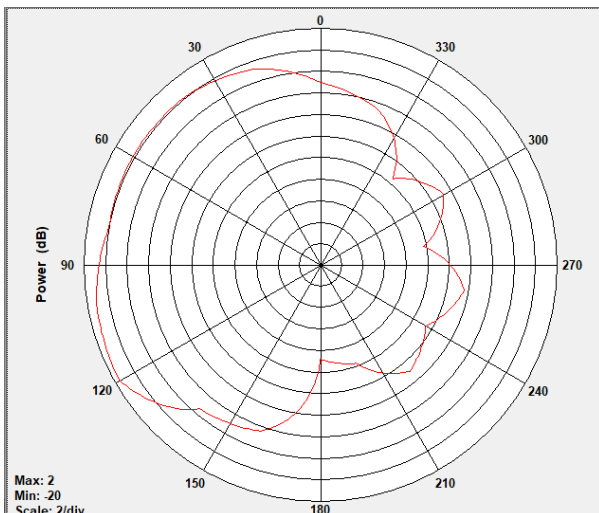
YZ-PLANE, f=2403\text{MHz}
