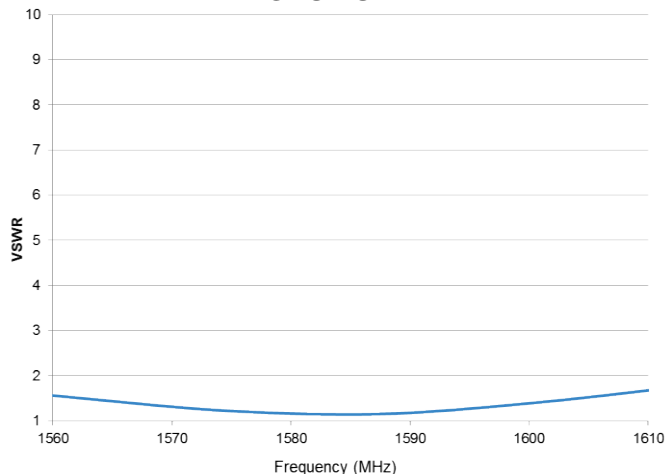
GPS VSWR
