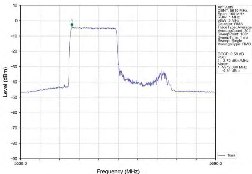
802.11ax(HEW80)_HCH_5610MHz_RU484_Left_Ant9_NTNV
