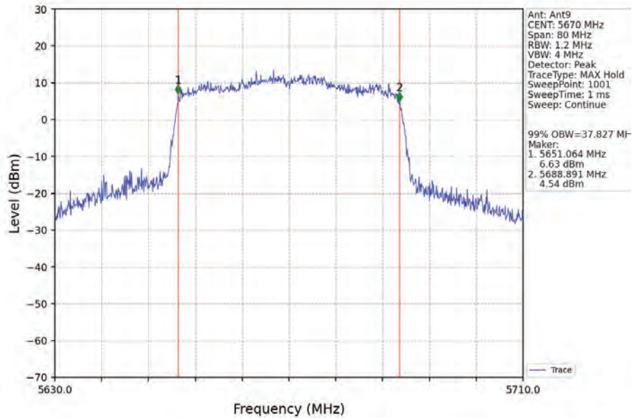
802.11ax(HEW40)_HCH_5670MHz_RU484_Left_Ant9_NTNV
