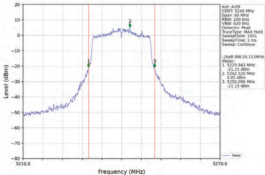
802.11n(HT20)_HCH_5240MHz_Ant9_NTNV
