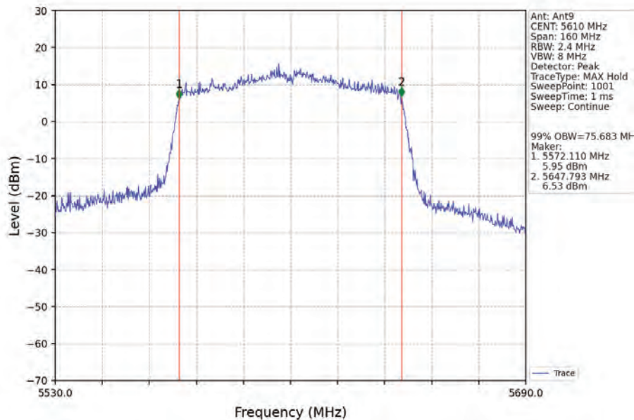
802.11ac(VHT80)_HCH_5610MHz_Ant9_NTNV
