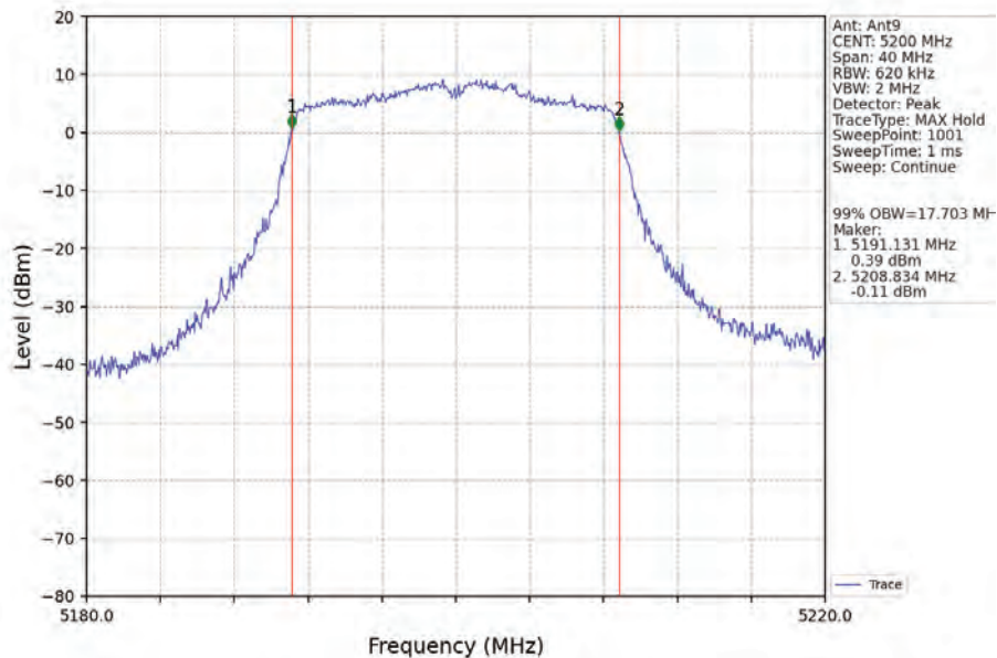
802.11n(HT20)_MCH_5200MHz_Ant9_NTNV
