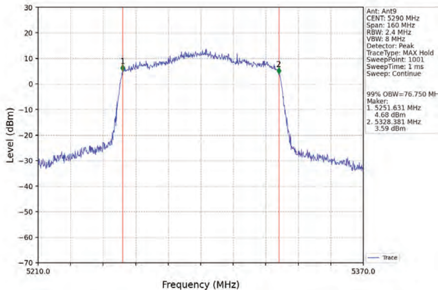
802.11ax(HEW80)_MCH_5290MHz_RU996_Left_Ant9_NTNV
