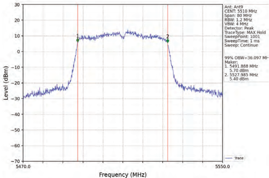
802.11ac(VHT40)_LCH_5510MHz_Ant9_NTNV
