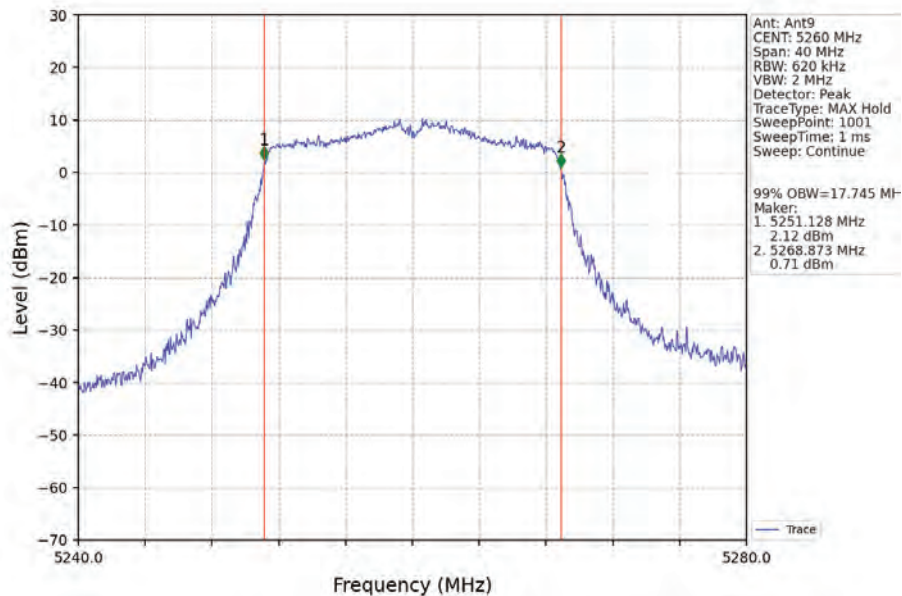
802.11n(HT20)_LCH_5260MHz_Ant9_NTNV
