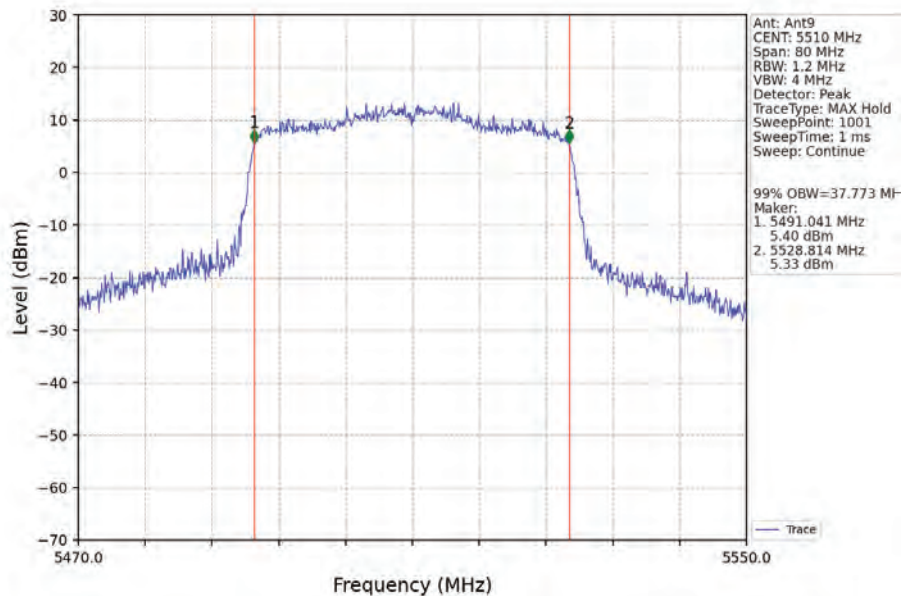
802.11ax(HEW40)_LCH_5510MHz_RU484_Left_Ant9_NTNV
