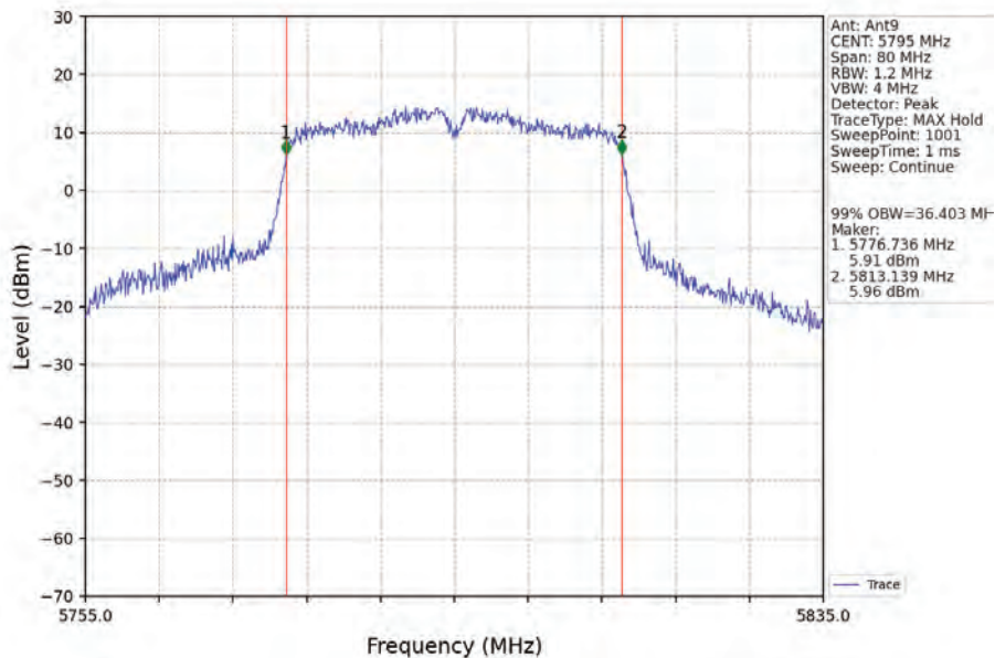
802.11ac(VHT40)_HCH_5795MHz_Ant9_NTNV
