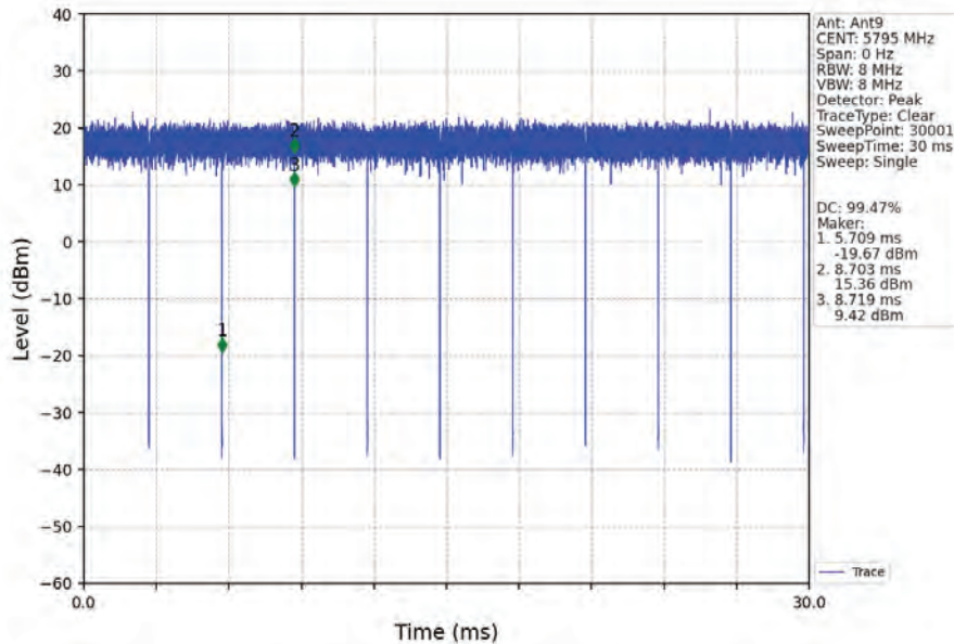
802.11ax(HEW40)_HCH_5795MHz_RU484_Left_Ant9_NTNV
