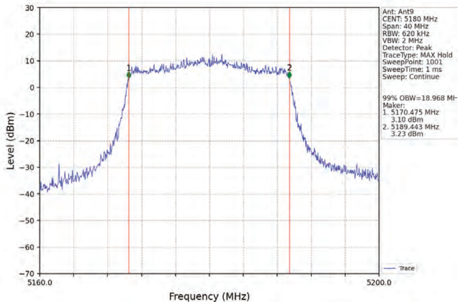
802.11ax(HEW20)_LCH_5180MHz_RU242_Left_Ant9_NTNV
