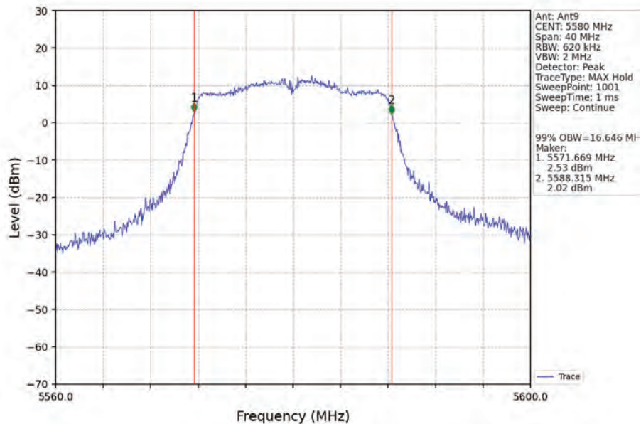
802.11a_MCH_5580MHz_Ant9_NTNV
