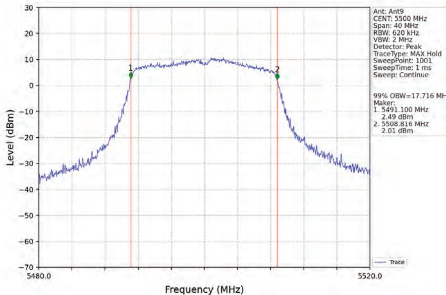
802.11ac(VHT20)_LCH_5500MHz_Ant9_NTNV
