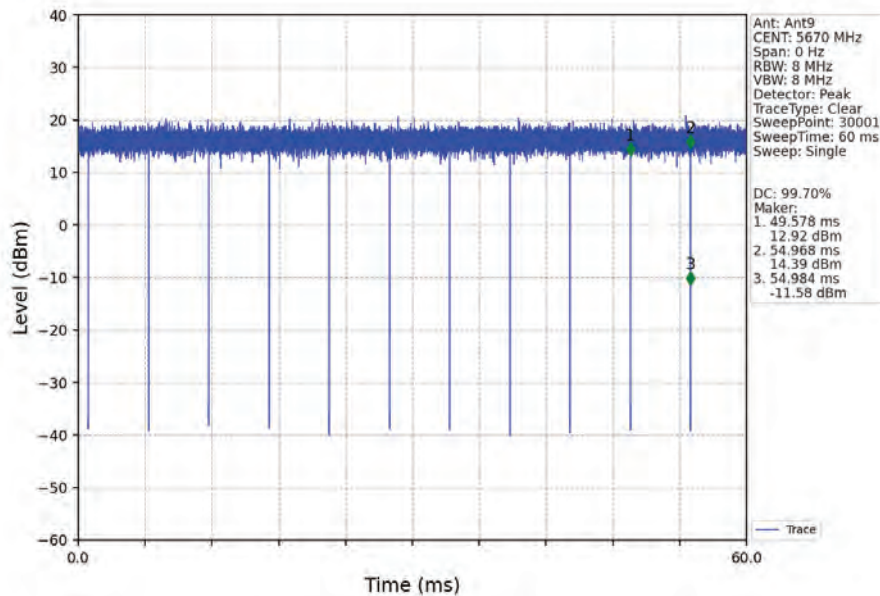
802.11ax(HEW40)_HCH_5670MHz_RU484_Left_Ant9_NTNV
