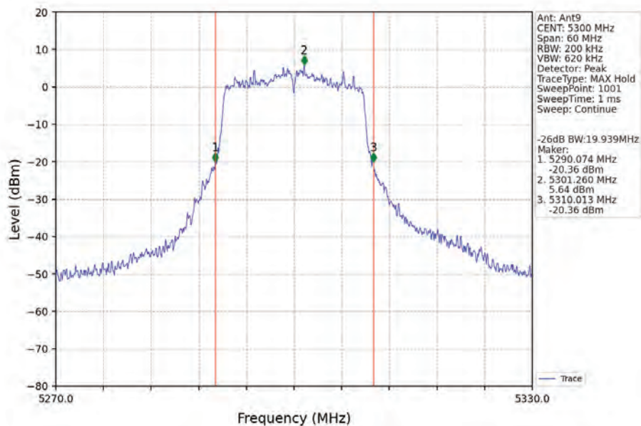
802.11n(HT20)_MCH_5300MHz_Ant9_NTNV
