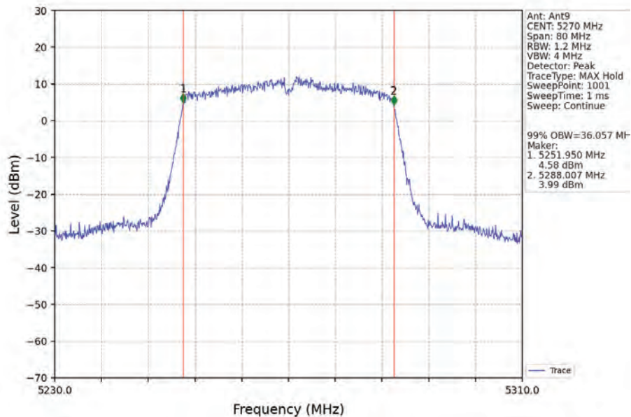
802.11ac(VHT40)_LCH_5270MHz_Ant9_NTNV
