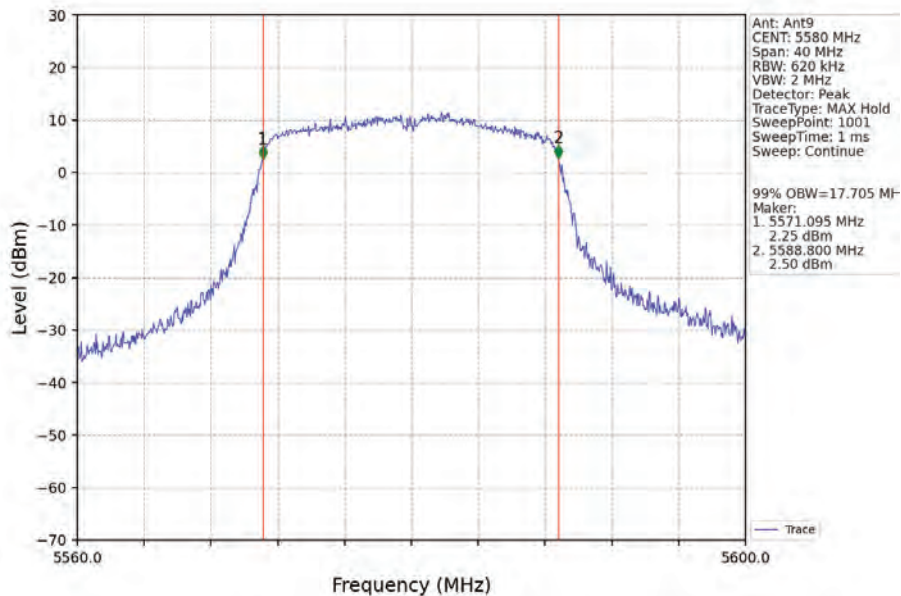
802.11n(HT20)_MCH_5580MHz_Ant9_NTNV
