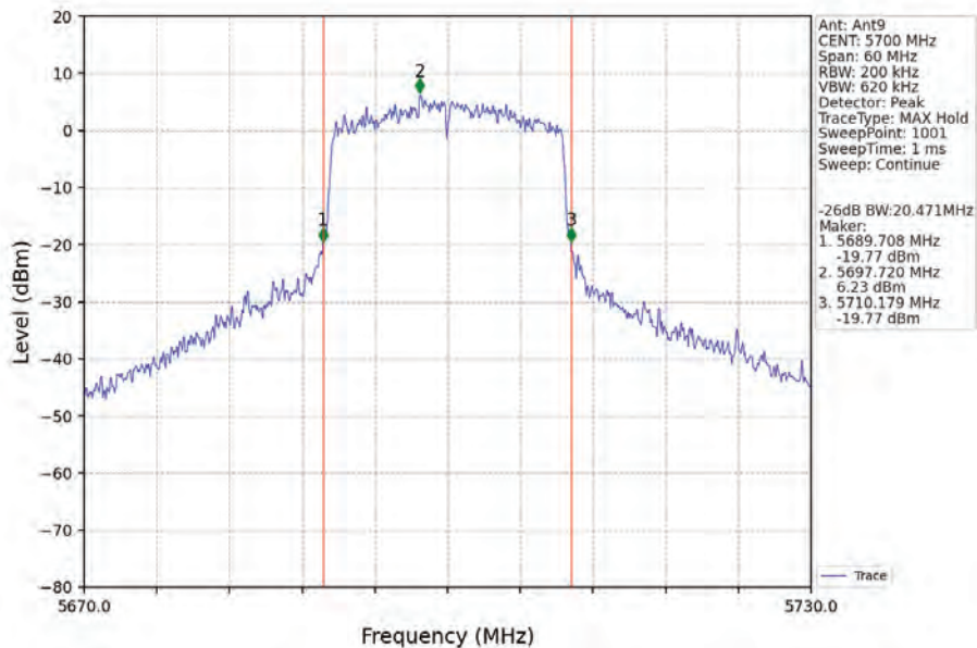
802.11ax(HEW20)_HCH_5700MHz_RU242_Left_Ant9_NTNV
