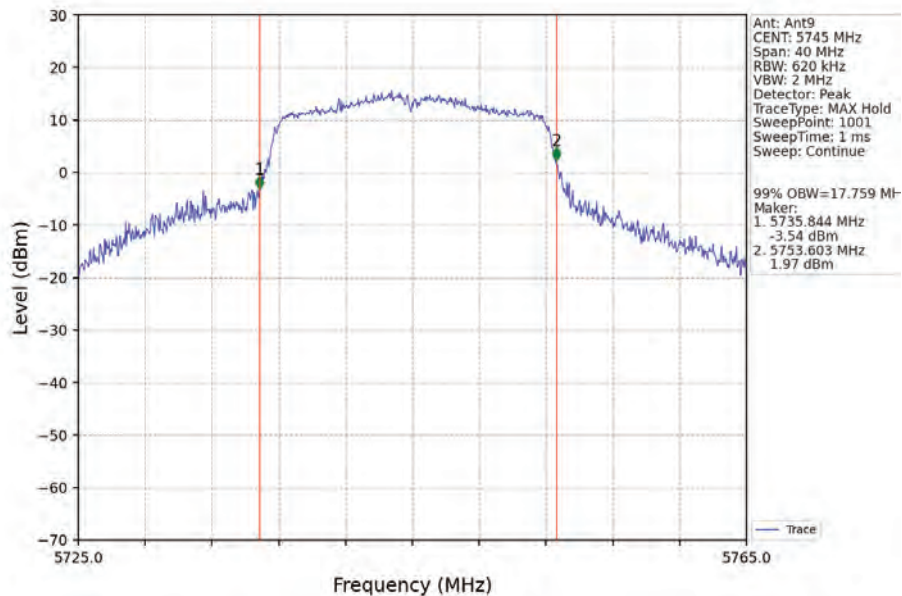
802.11a_LCH_5745MHz_Ant9_NTNV
