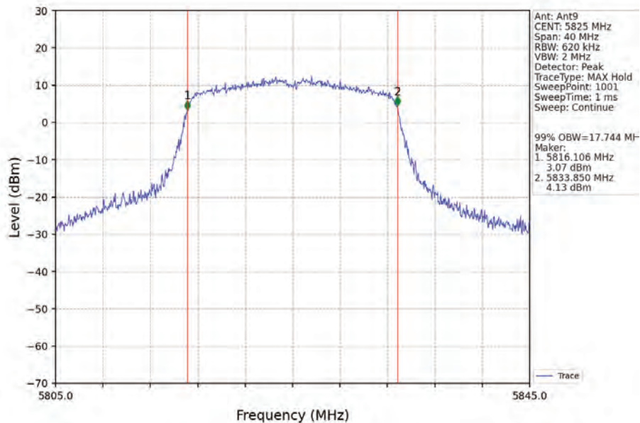
802.11n(HT20)_HCH_5825MHz_Ant9_NTNV
