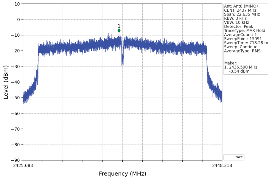
802.11ax(HEW20)_MCH_2437MHz_RU242_Left_Ant8 (MIMO)_NTNV
