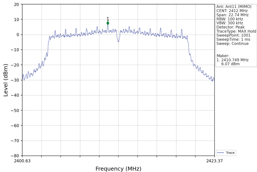
802.11g_LCH_2412MHz_Ant11 (MIMO)_NTNV
