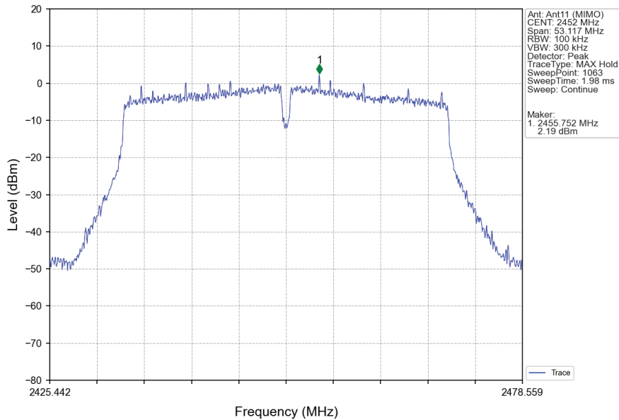
802.11n(HT40)_HCH_2452MHz_Ant11 (MIMO)_NTNV
