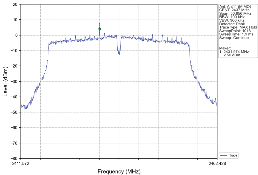
802.11n(HT40)_MCH_2437MHz_Ant11 (MIMO)_NTNV
