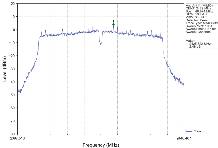
802.11n(HT40)_LCH_2422MHz_Ant11 (MIMO)_NTNV
