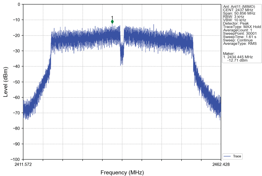
802.11n(HT40)_MCH_2437MHz_Ant11 (MIMO)_NTNV
