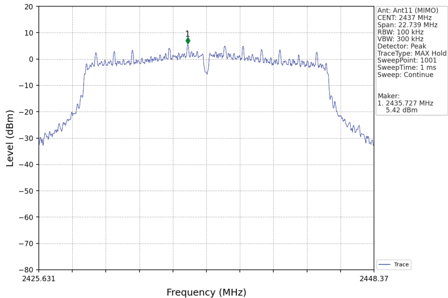
802.11g_MCH_2437MHz_Ant11 (MIMO)_NTNV
