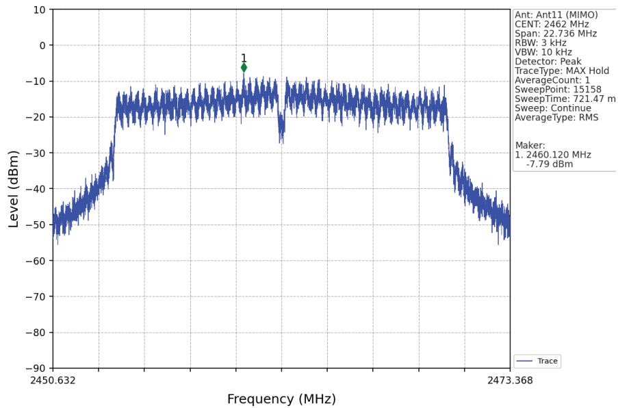
802.11g_HCH_2462MHz_MIMO_NTNV
