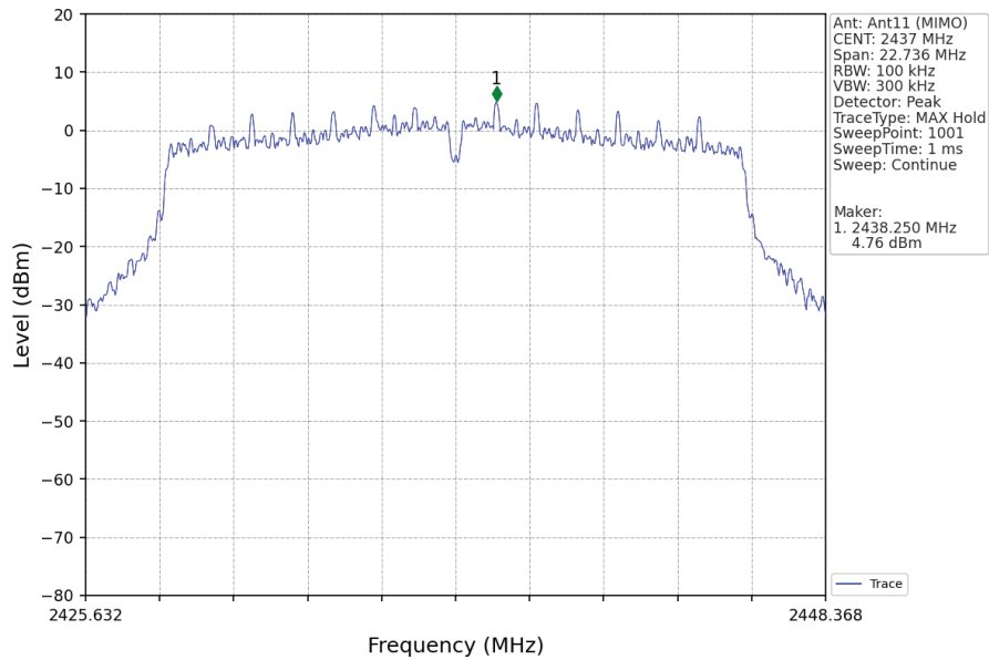
802.11n(HT20)_MCH_2437MHz_Ant11 (MIMO)_NTNV
