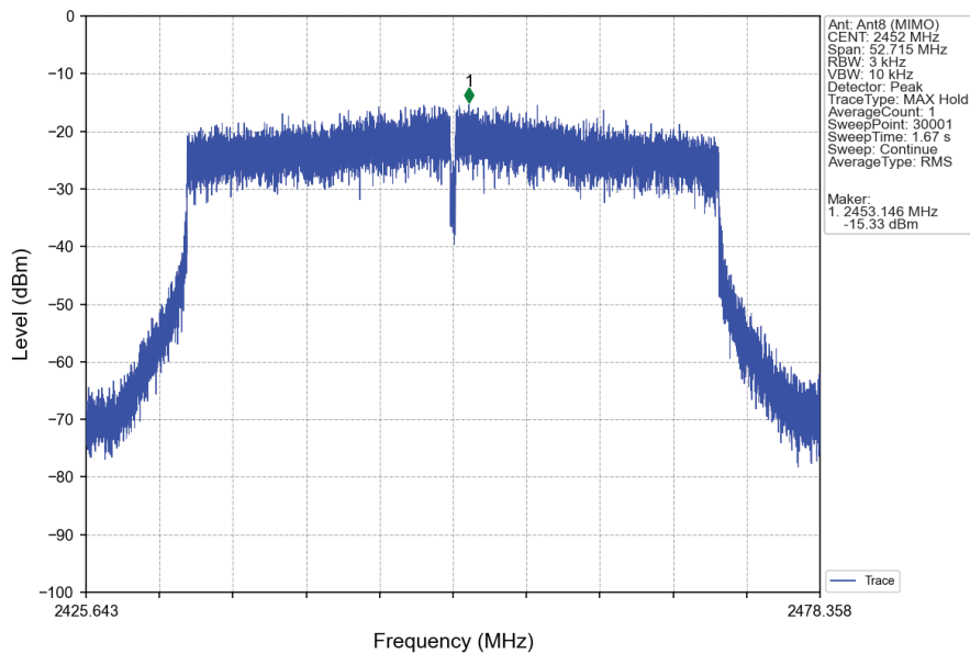
802.11ax(HEW40)_HCH_2452MHz_RU484_Left_Ant8 (MIMO)_NTNV
