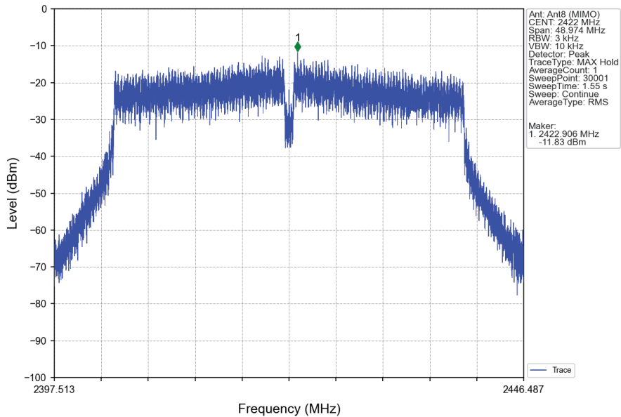
802.11n(HT40)_LCH_2422MHz_Ant8 (MIMO)_NTNV
