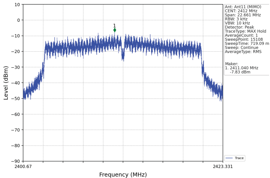
802.11n(HT20)_LCH_2412MHz_Ant11 (MIMO)_NTNV
