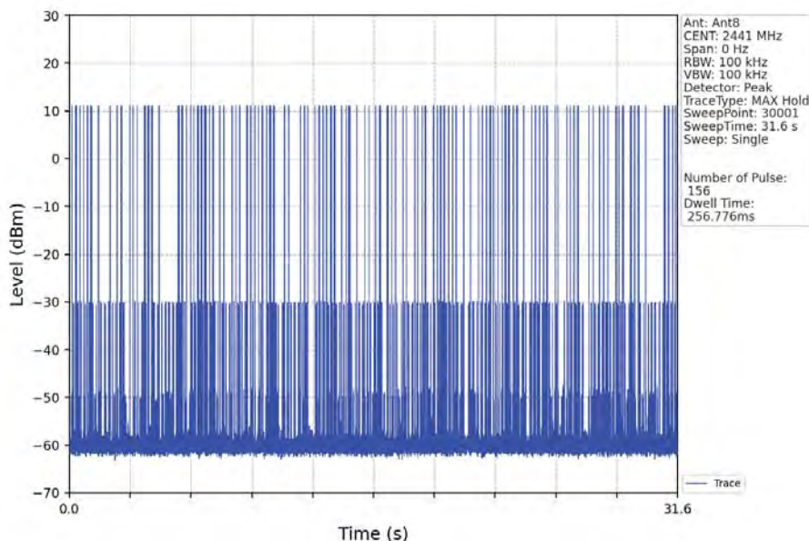
Pi/4DQPSK_2DH3_HOPP_Ant8_NTNV
