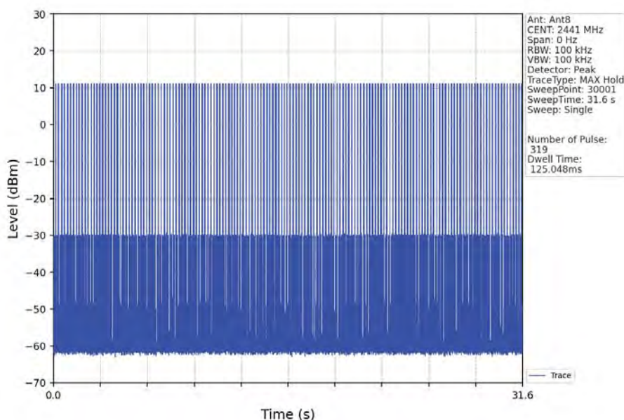
Pi/4DQPSK_2DH1_HOPP_Ant8_NTNV
