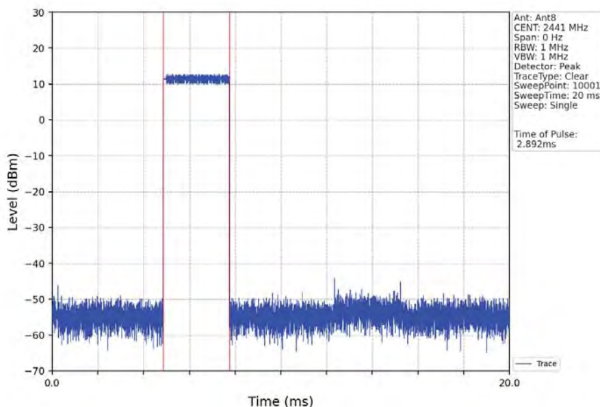
Pi/4DQPSK_2DH5_HOPP_Ant8_NTNV
