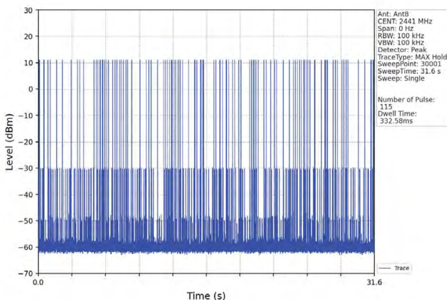
Pi/4DQPSK_2DH5_HOPP_Ant8_NTNV
