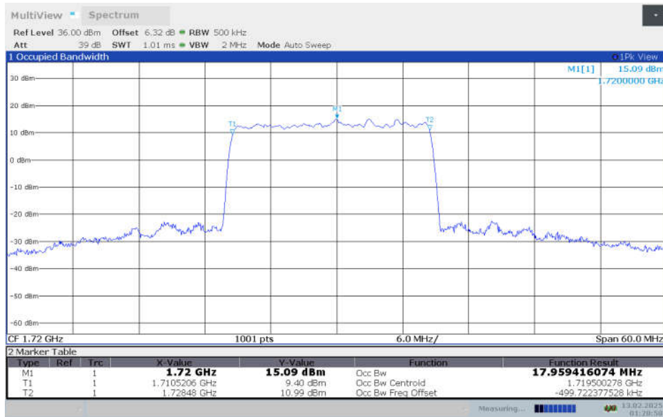
n66,20MHz Bandwidth,CP-QPSK (99% OBW)
