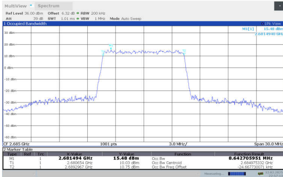
n41,10MHz Bandwidth,CP-QPSK (99% OBW)
