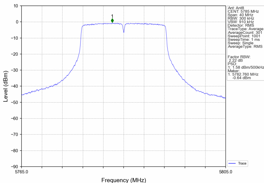
802.11a MCH 5785MHz Ant8 NTN
