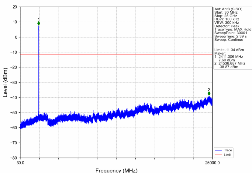
802.11b_LCH_2412MHz_Ant8 (SISO)_NTNV
